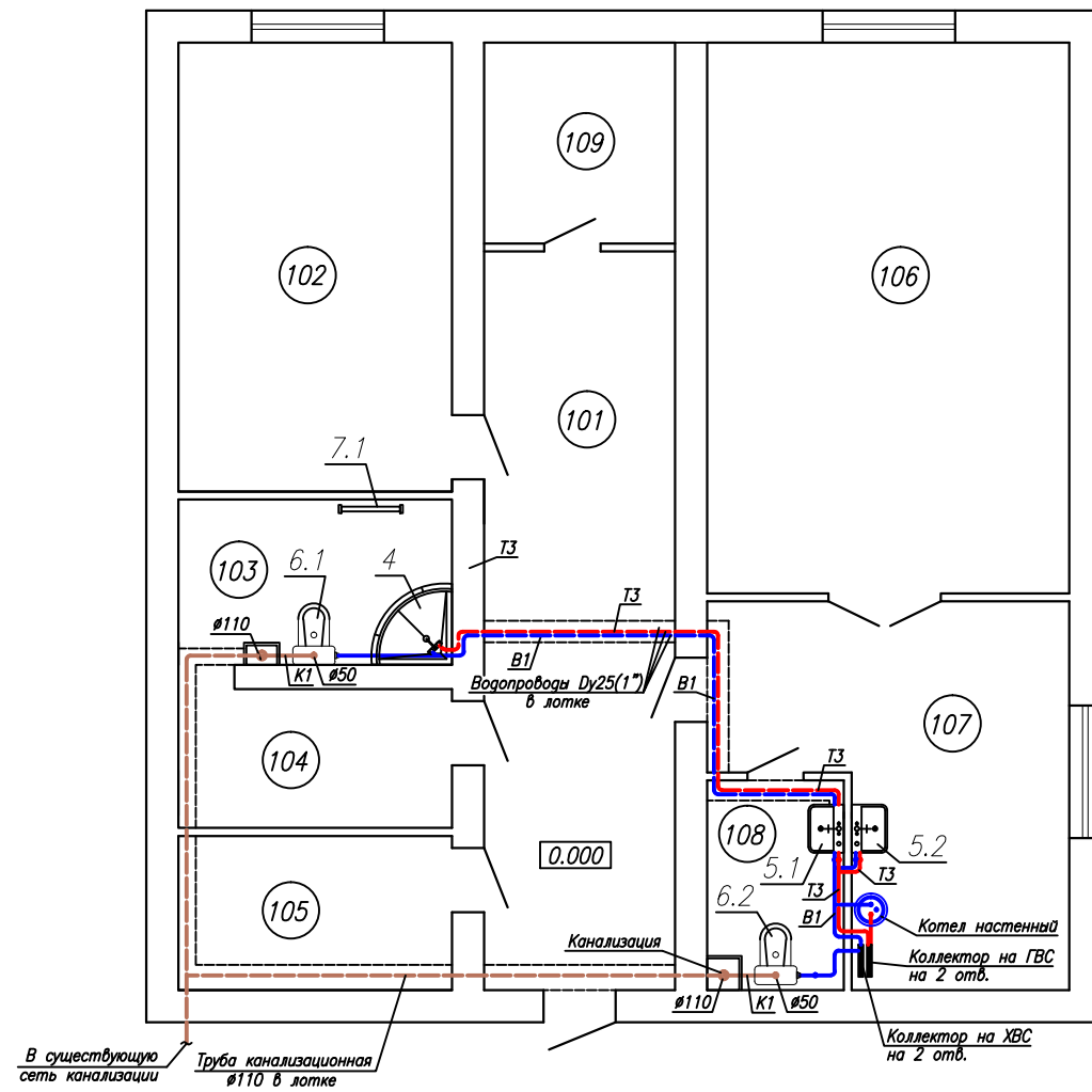
План 1-го этажа (1:100)
