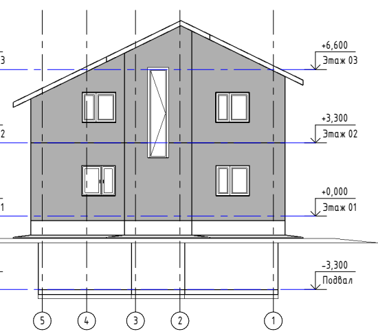
В_АР_Ф_Северный
