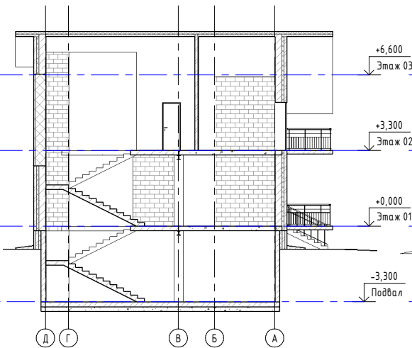
Разрез 1
