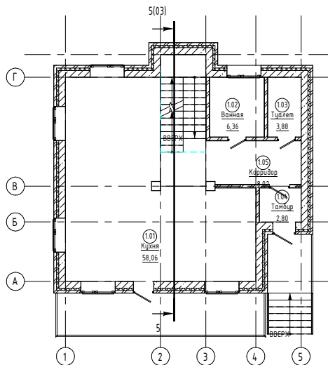
В_АР_ПЭ_01 Этаж
