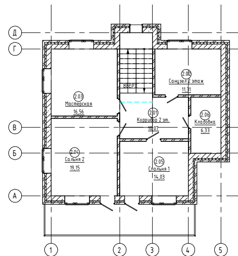
В_АР_ПЭ_02 Этаж
