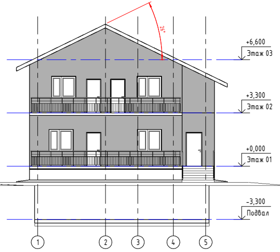
В_АР_Ф_Южный
