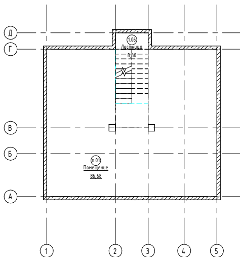
В_АР_ПЭ_Подвал
