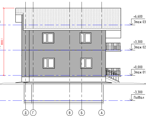
В_АР_Ф_Западный
