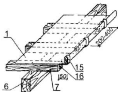
Рисунок 3.9. Крепление фронтового края рядовой полосы
