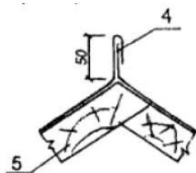
Рисунок 3.8. Коньковый гребневый фальц 4 - коньковый гребневый фальц; 5 - доска
