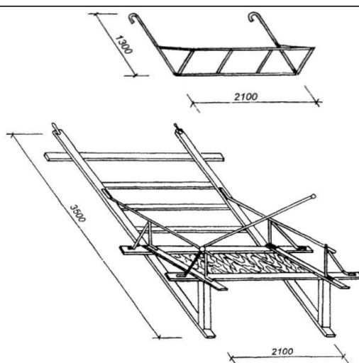
Рисунок 3.4. Инвентарная сборно-разборная площадка и металлическая подставка
