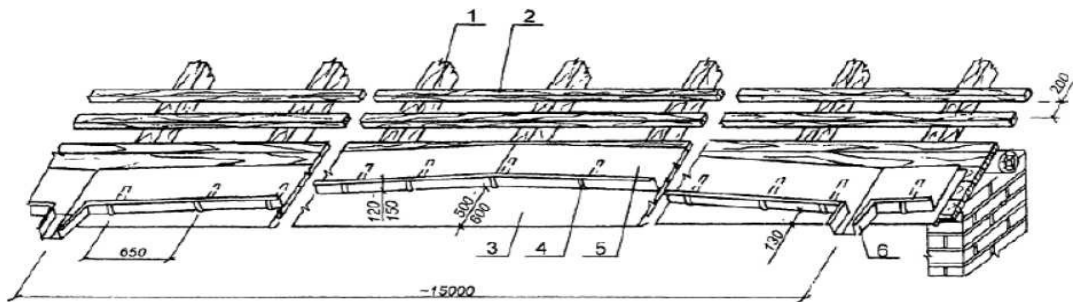
Рисунок 3.6. Схема укладки настенных желобов
