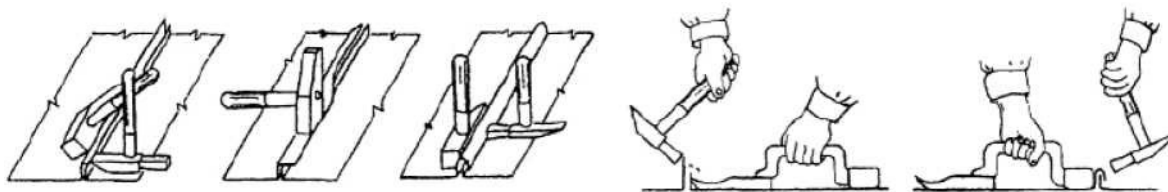
Рисунок 3.13. Соединение картин гребневым фальцем с помощью молотка и бруса-отворотки.
