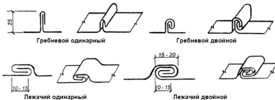
Рисунок 3.3. Виды фальцев
