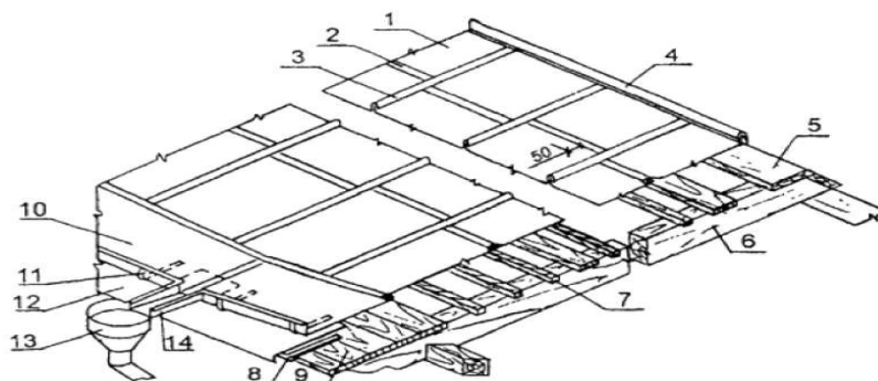
Рисунок 3.7. Схема устройства кровли из листовой стали
