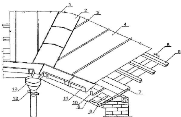
Рисунок 3.11. Схема устройства разжелобка
