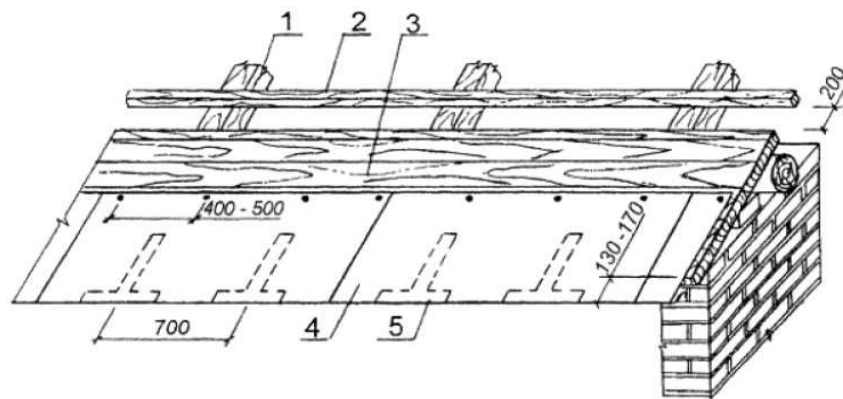
Рисунок 3.5. Схема устройства карнизного свеса
