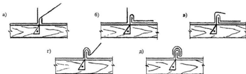
Рисунок 3.10. Схема соединения листов стоячим фальцем с креплением их кляммерой к обрешётке
