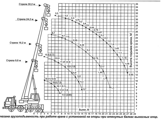
Рисунок 2.1. Грузовые характеристики автомобильного стрелового крана КС-55729-5В
