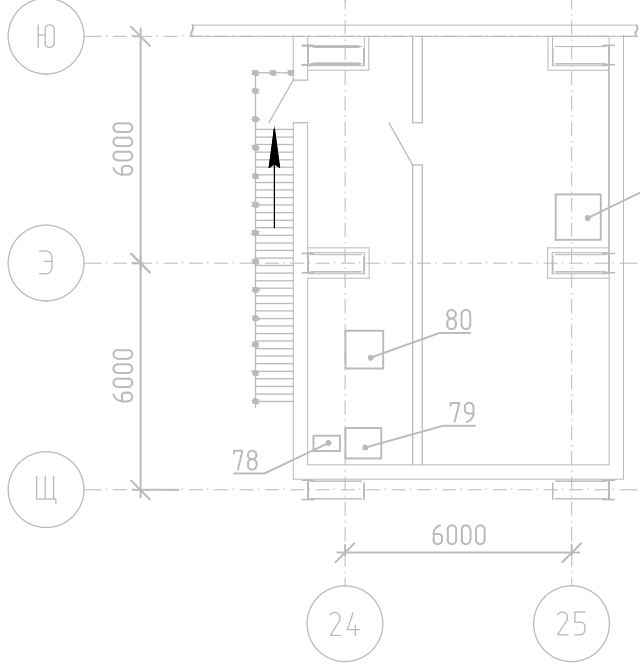
План химической лаборатории на отм. +4,00 в осях Щ-Ю/24-25
