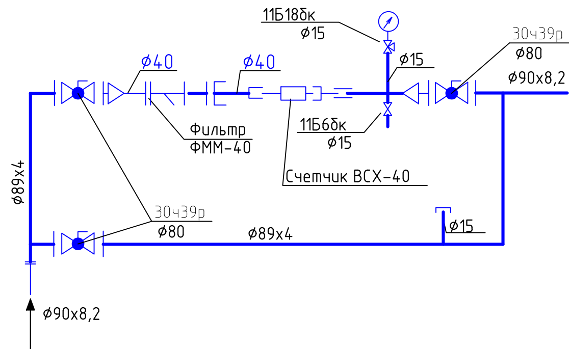
Водомерный узел со счетчиком ВСХ-40
