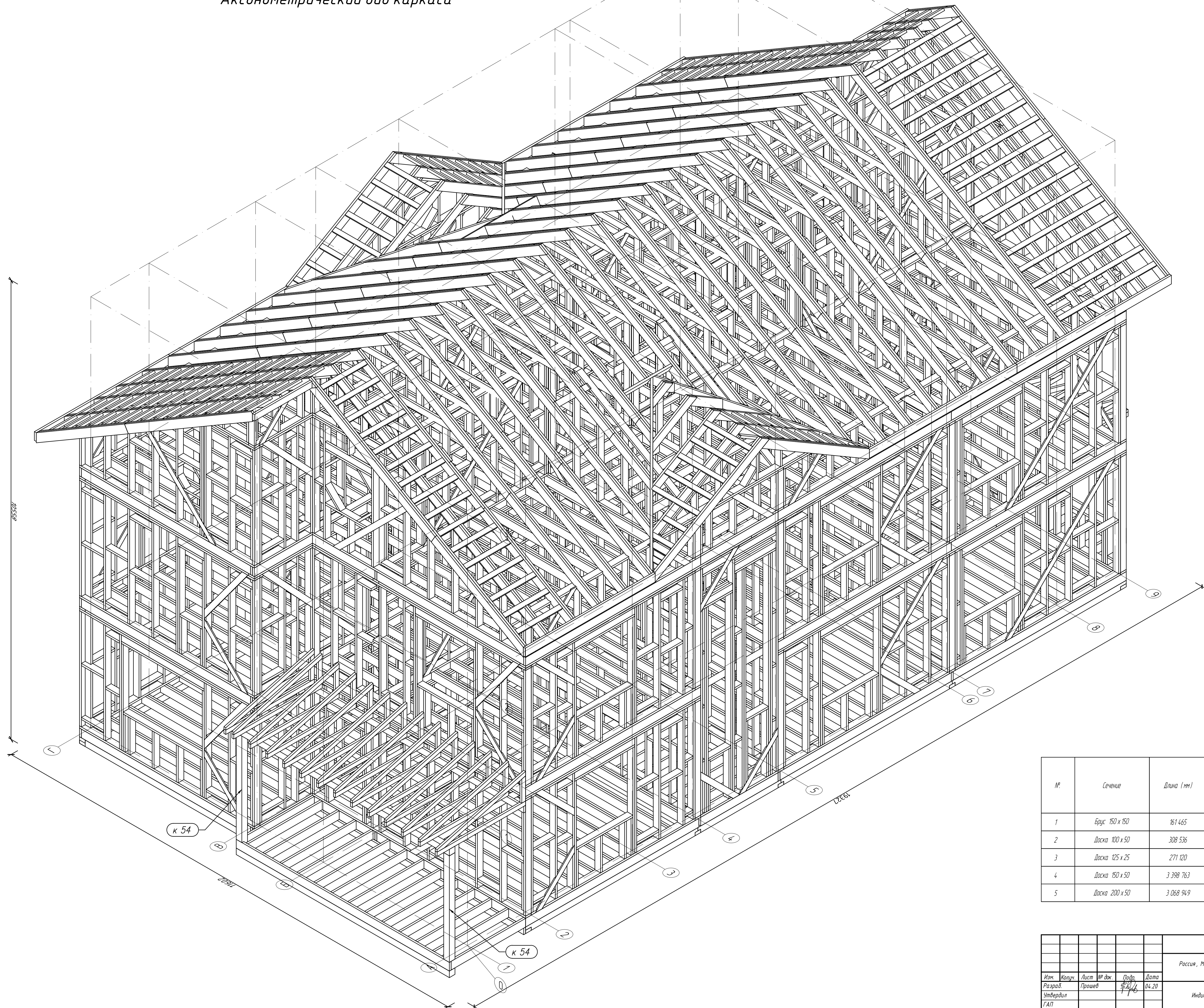
Аксонетрический вид каркаса
