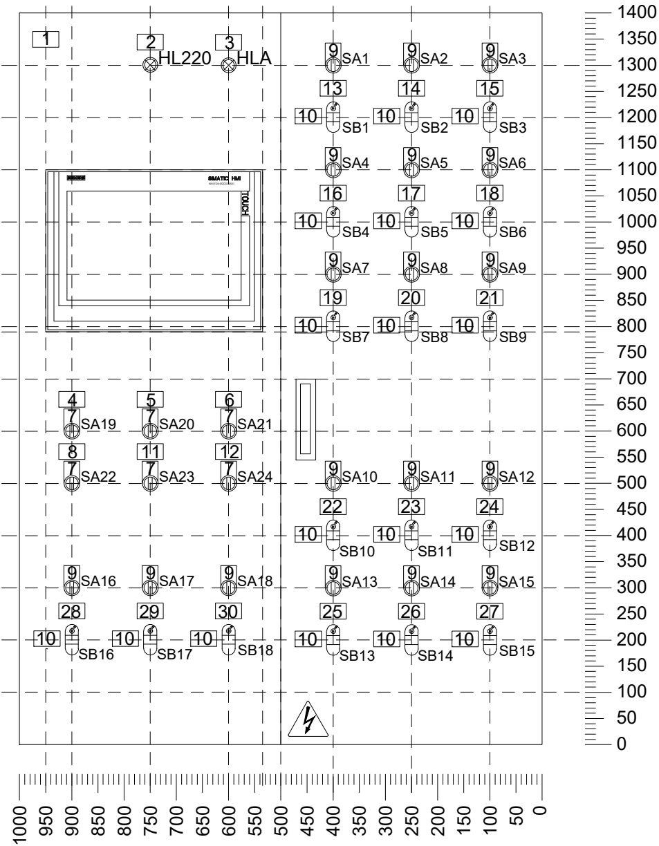
Шкаф ШАОК. Вид спереди (дверь щита)
