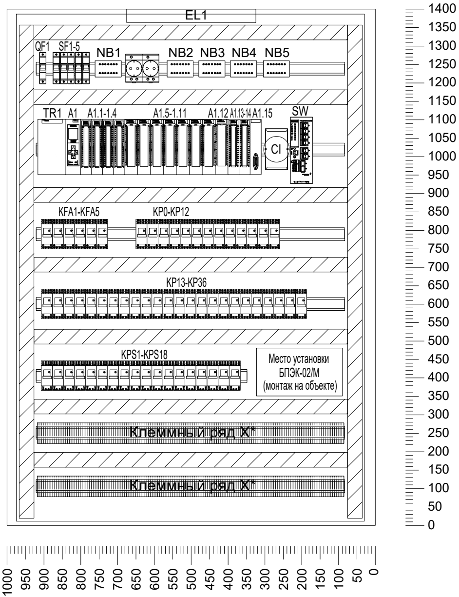
Шкаф ШАОК. Вид спереди (дверь щита условно не показана)
