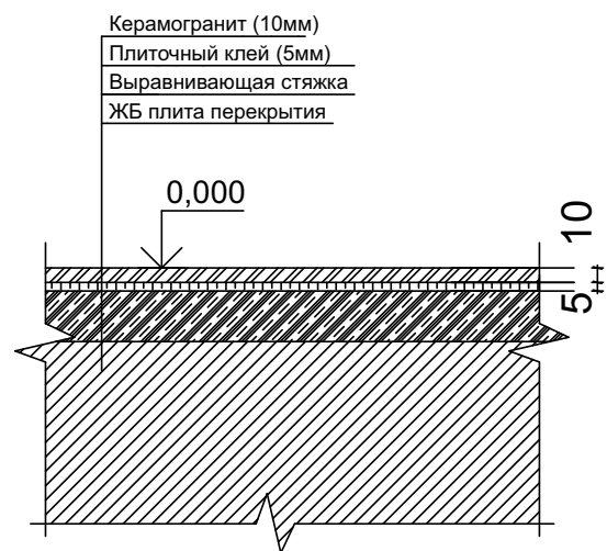
Тип пола А-02
