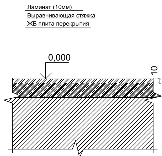
Тип пола А-04
