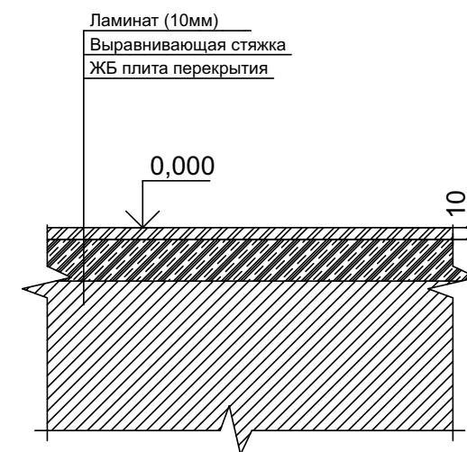
Тип пола А-03
