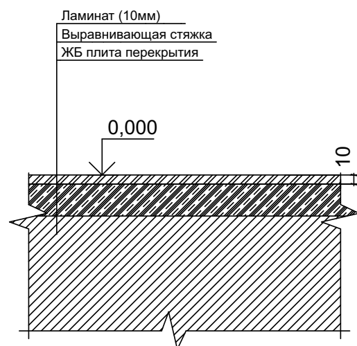
Тип пола А-05
