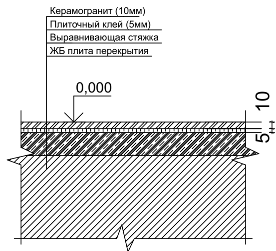
Тип пола А-01
