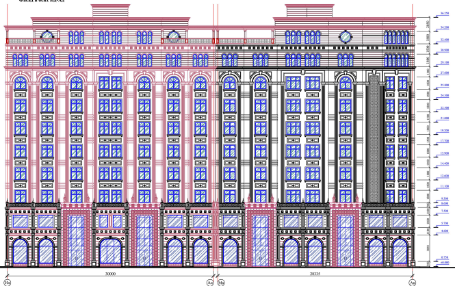
Фасад в осях Пд-Ад
