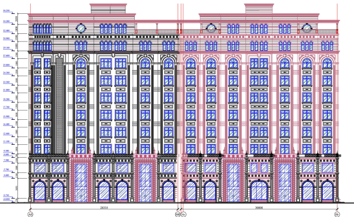
Фасад в осях А6-М6
