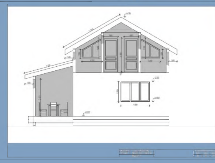
Проектное решение после внесения изменений
