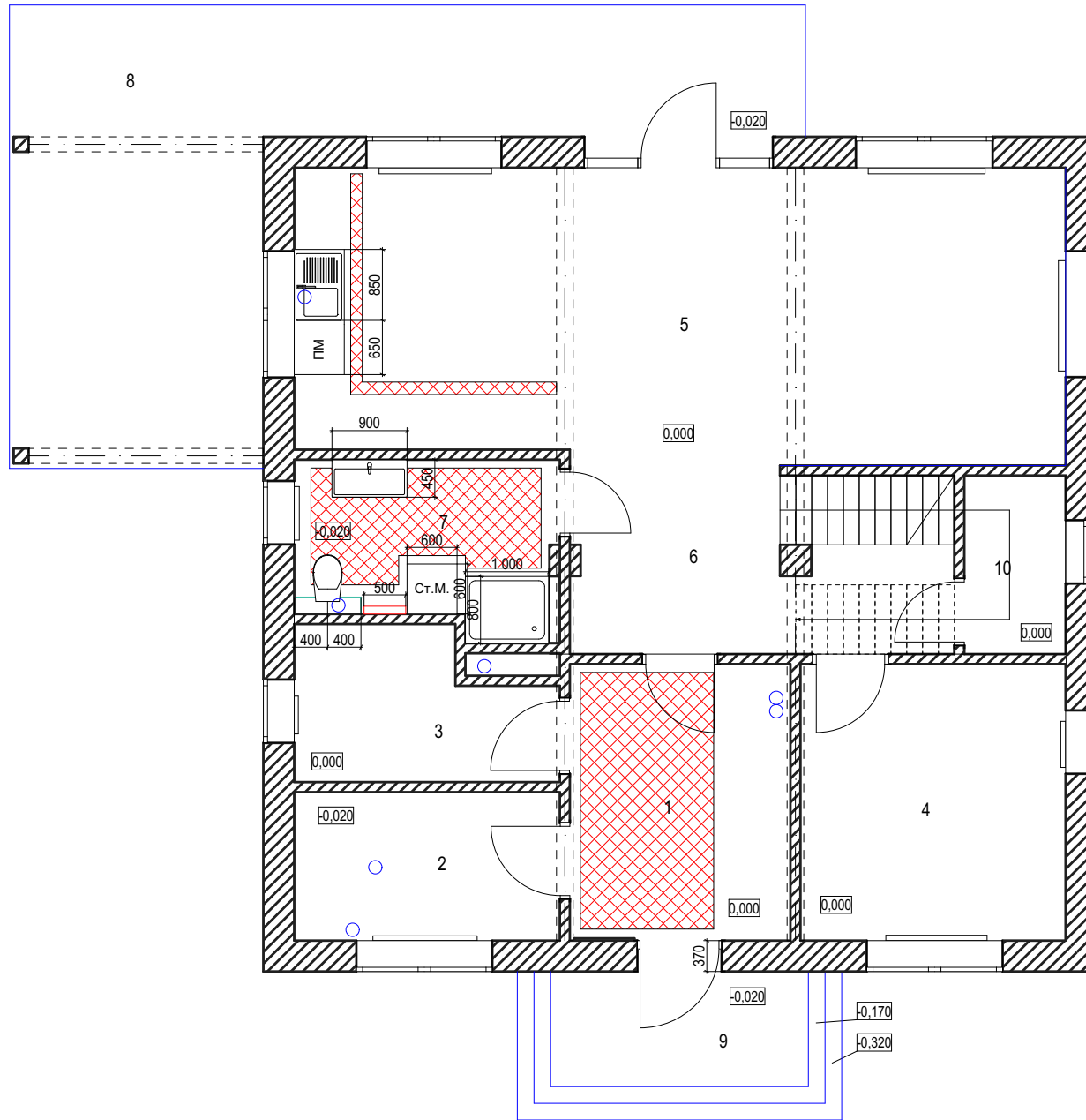
План установки теплых полов и сантехники 1 этаж
