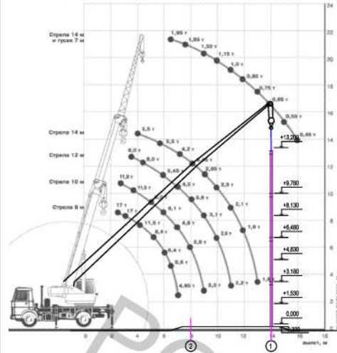
Схема монтажа колонн вдоль оси "1" М1:200
