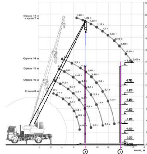
Схема монтажа колонн вдоль оси "2" М1:200
