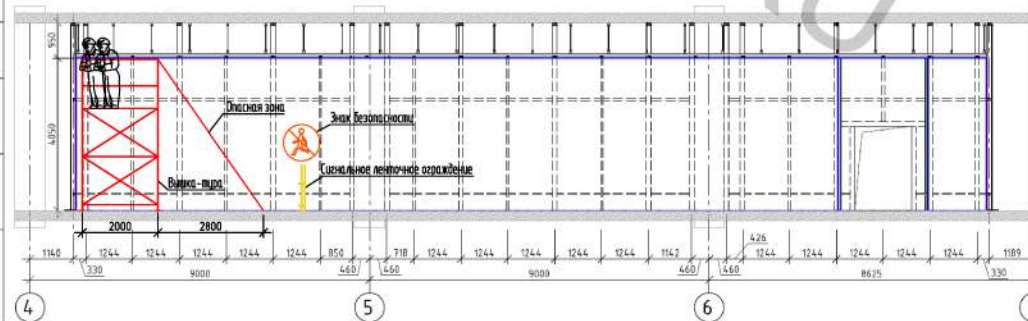
Разрез 1-1 М1:100
