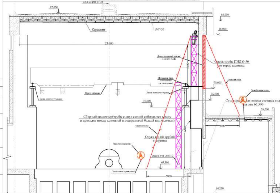
Схема демонтажа витража нижнего бьефа
