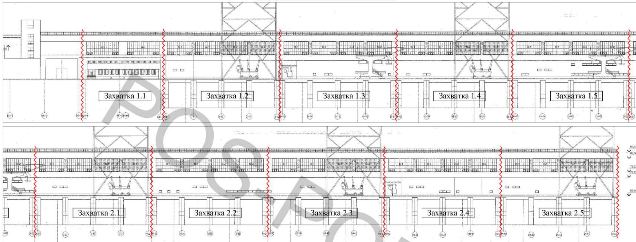
Схема демонтажа витража нижнего бьефа
