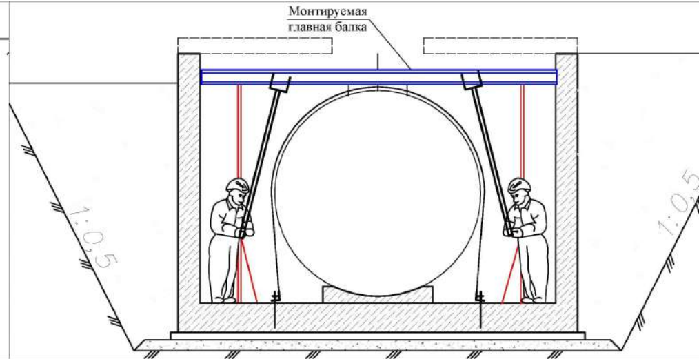
Этап 2. Монтаж главных балок
