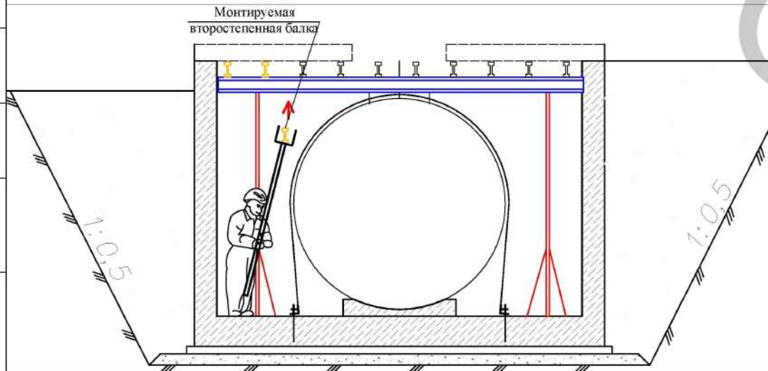
Этап 3. Монтаж второстепенных балок
