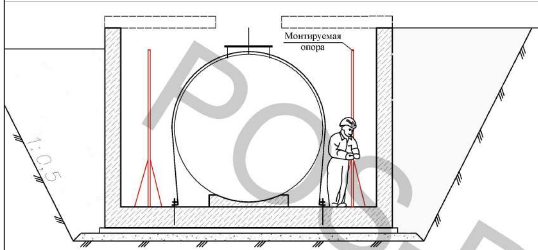
Этап 1. Установка опор
