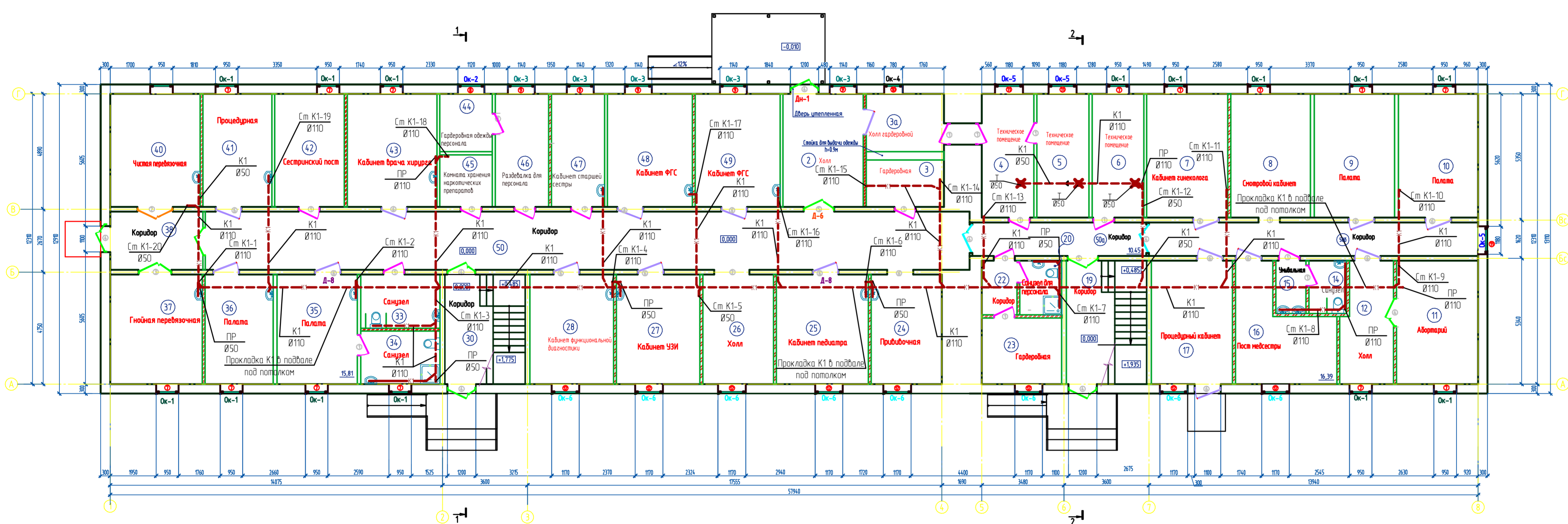
План 1-ого этажа после капитального ремонта
