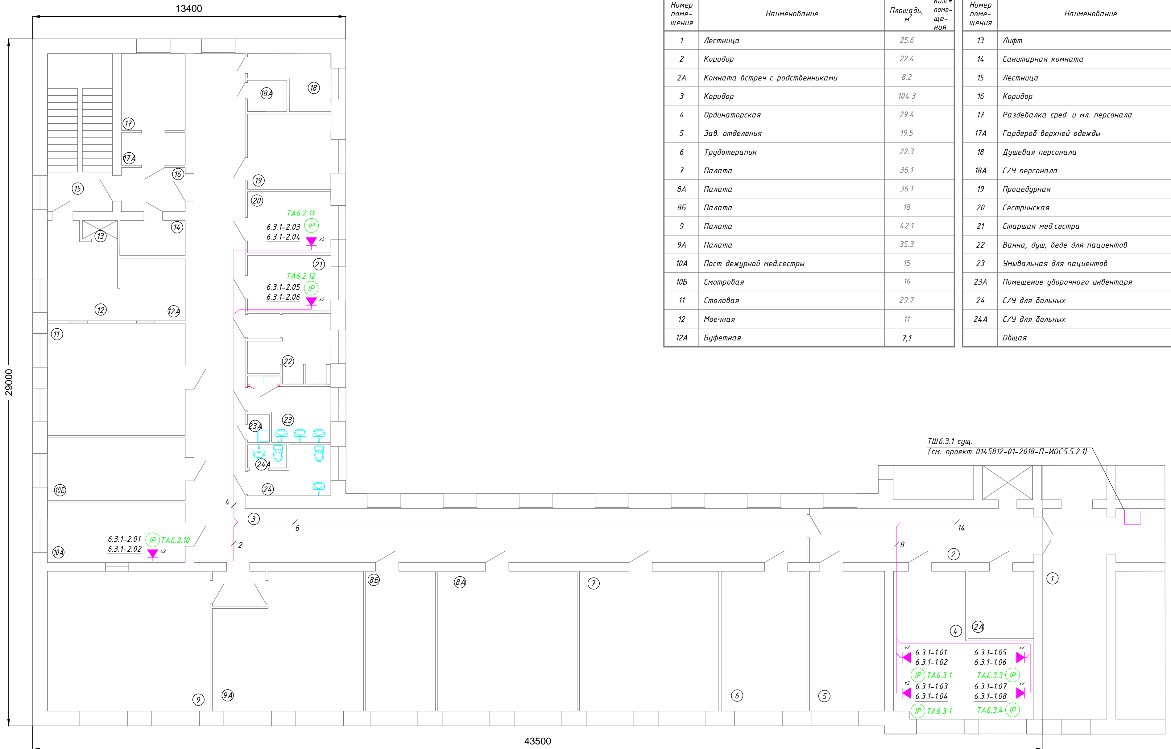
Фрагмент плана 3-го этажа
