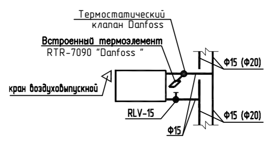
5 Подключение радиатора с длиной менее 1400 мм
