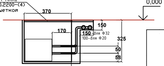
Разрез 1-1.
