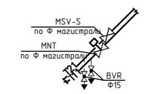
2 Расположение балансировочных клапанов на горизонтальных магистральных
