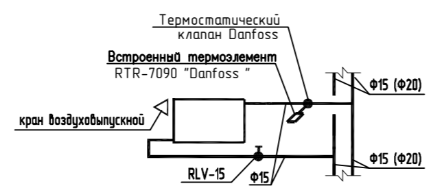
4 Подключение радиатора с длиной 1400 мм и более
