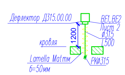
Схема ВЕ1, ВЕ2
