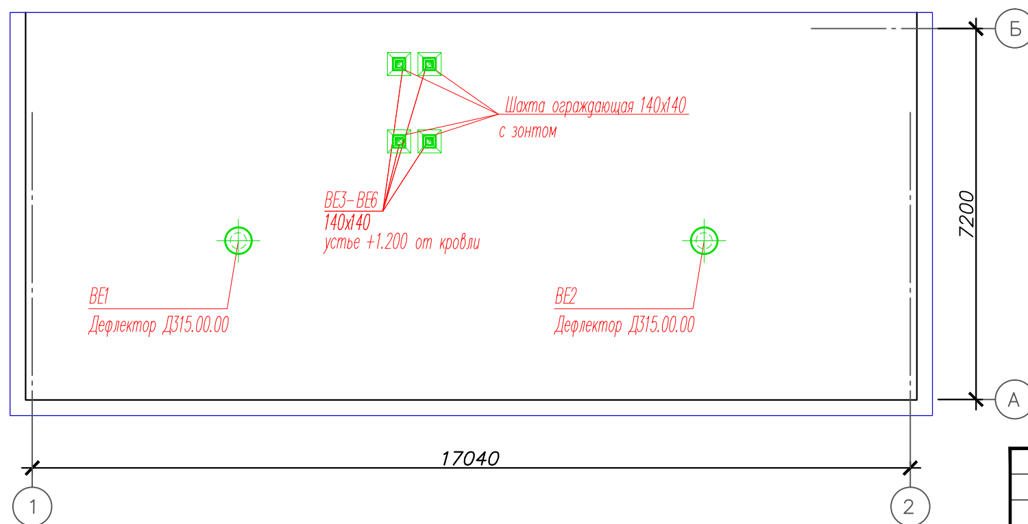
План шахты.
