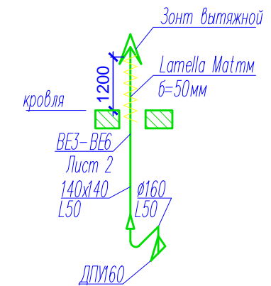
Схема ВЕ3-ВЕ6
