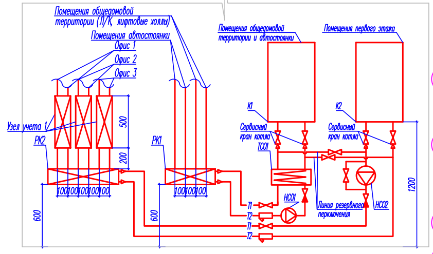
Схема узла управления системой отопления
