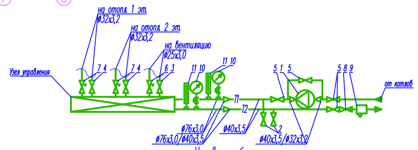
Схема узла управления
