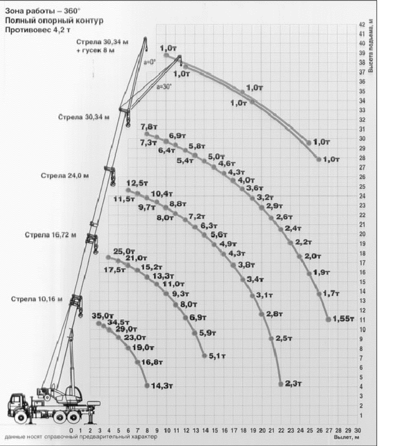
Грузовысотные характеристики автокрана КС-55735-7 грузоподъемностью 35 т на шасси КАМАЗ
