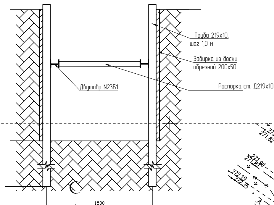
Устройство траншеи
