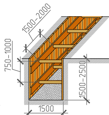
Устройство траншеи
