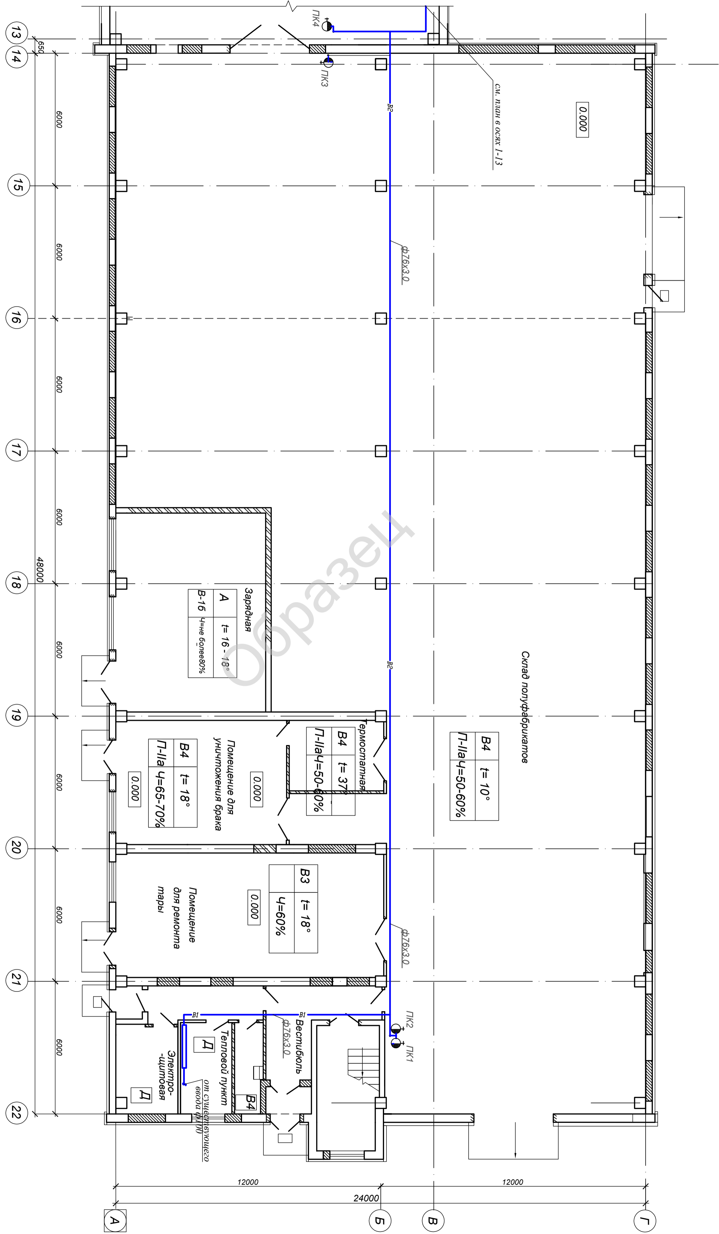
План на стп. 0.000
