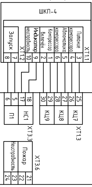
Компрессор
