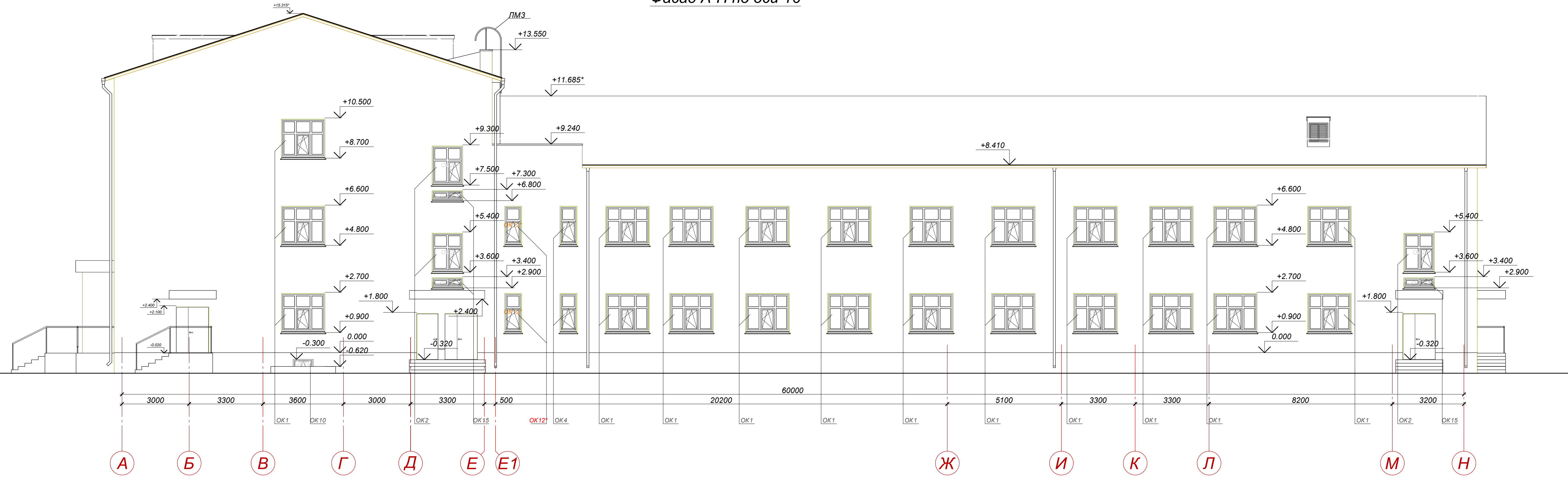
Фасад А-Н по оси 16
