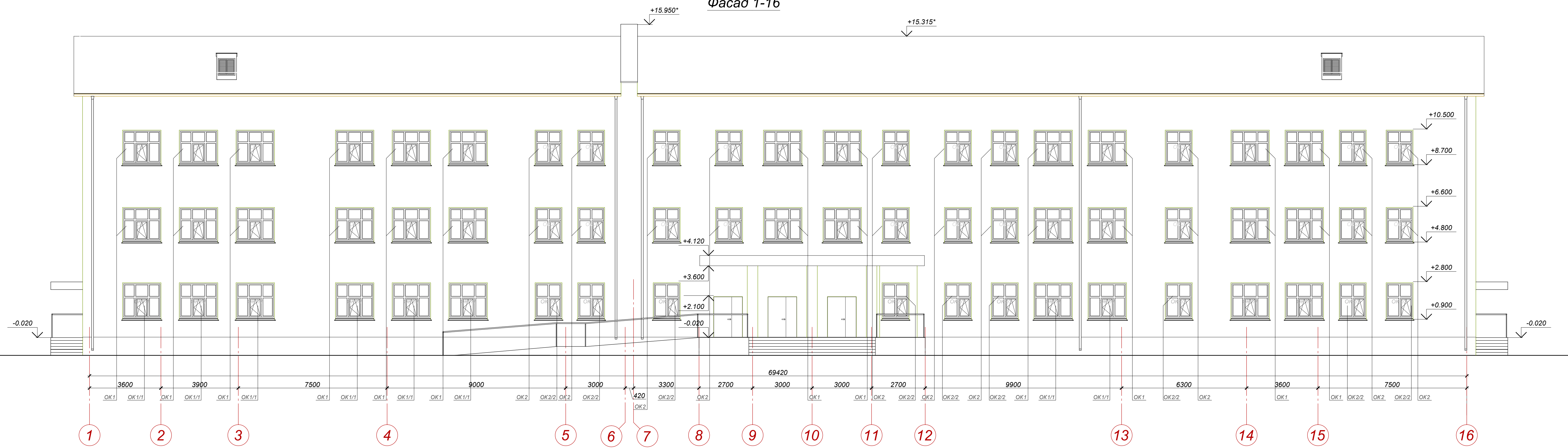
Фасад 1-16
