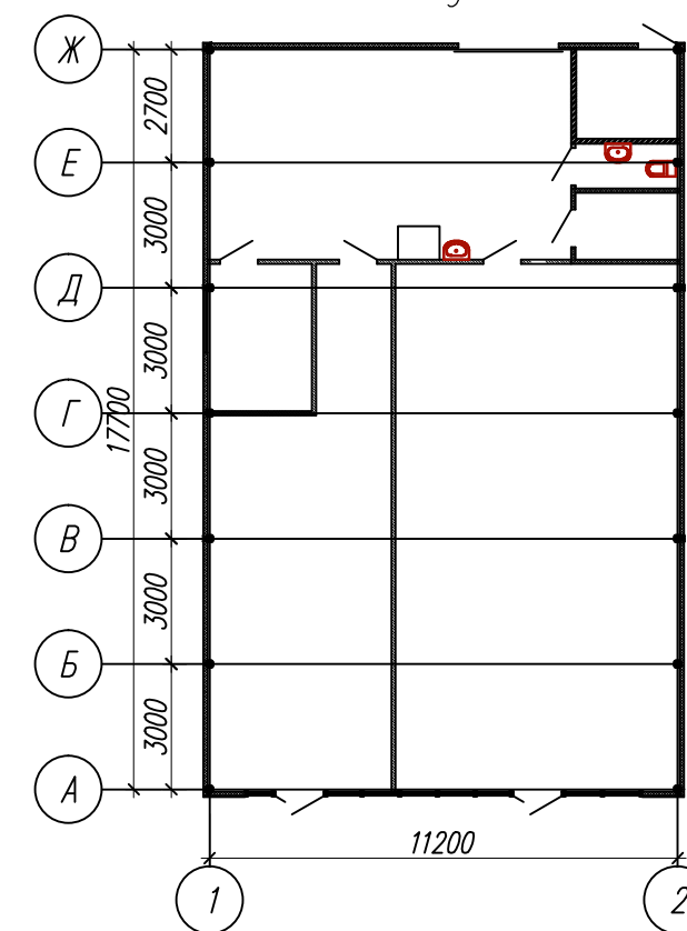
План здания.
