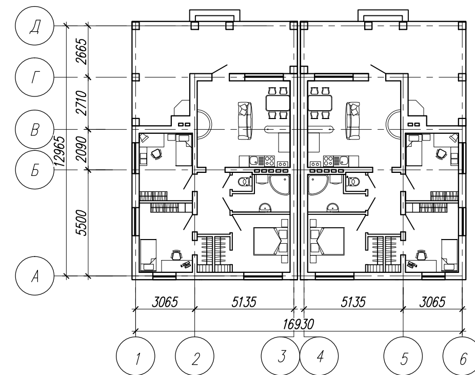
План здания.
