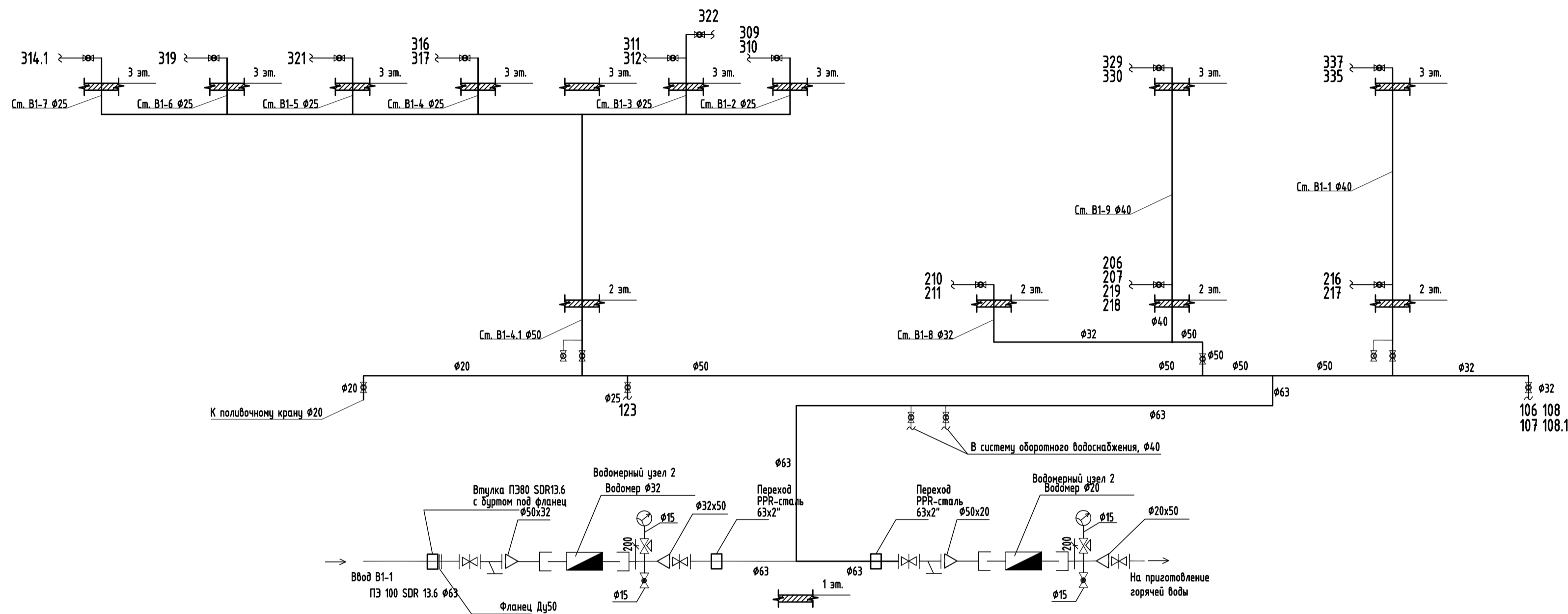
Принципиальная схема системы В1
