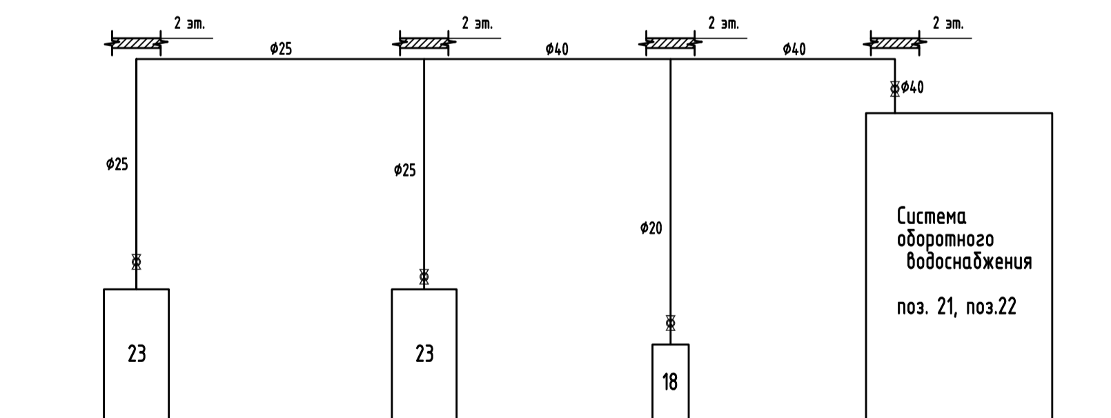
Принципиальная схема системы В4
