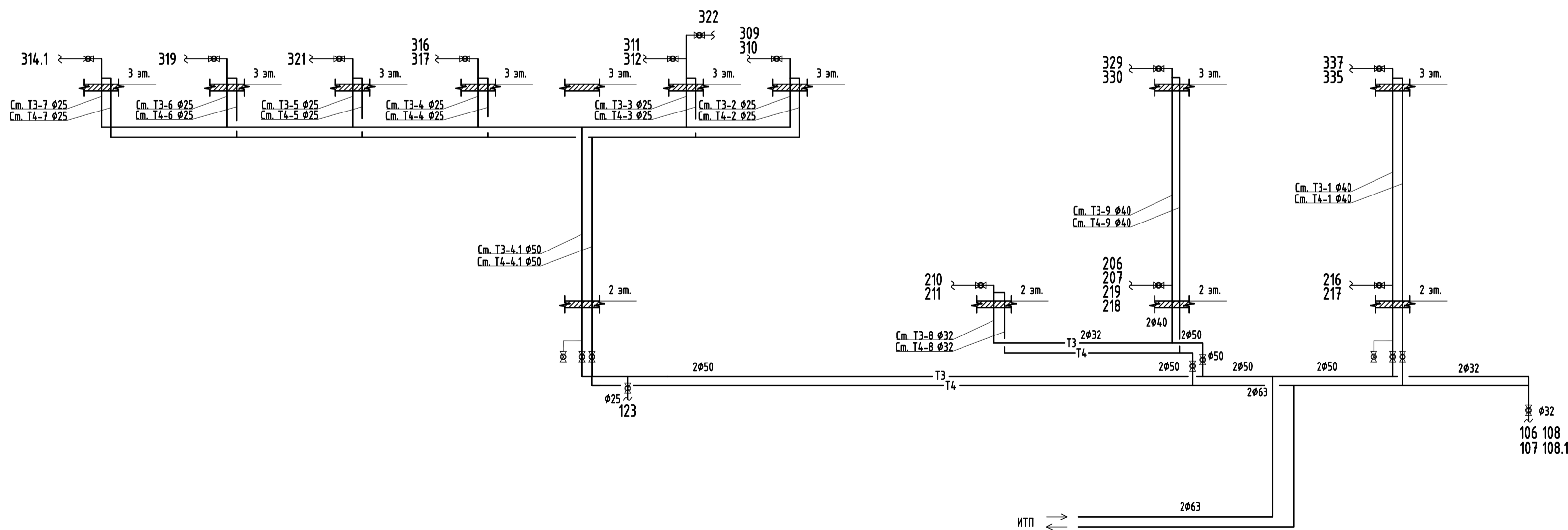
Принципиальная схема системы Т3, Т4
