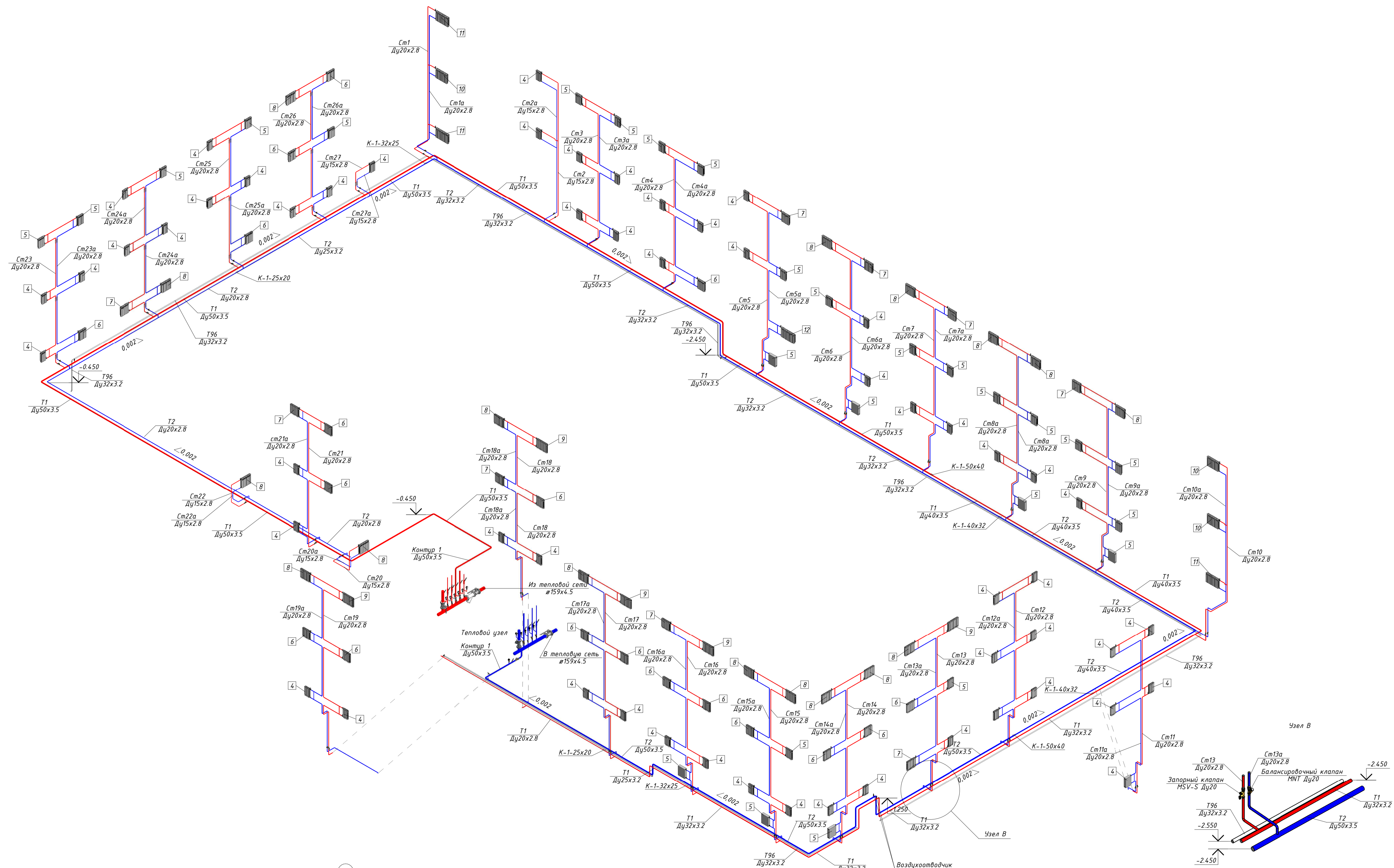
АксонOMETрический вид системы отопления в осях 7-20/М-У
