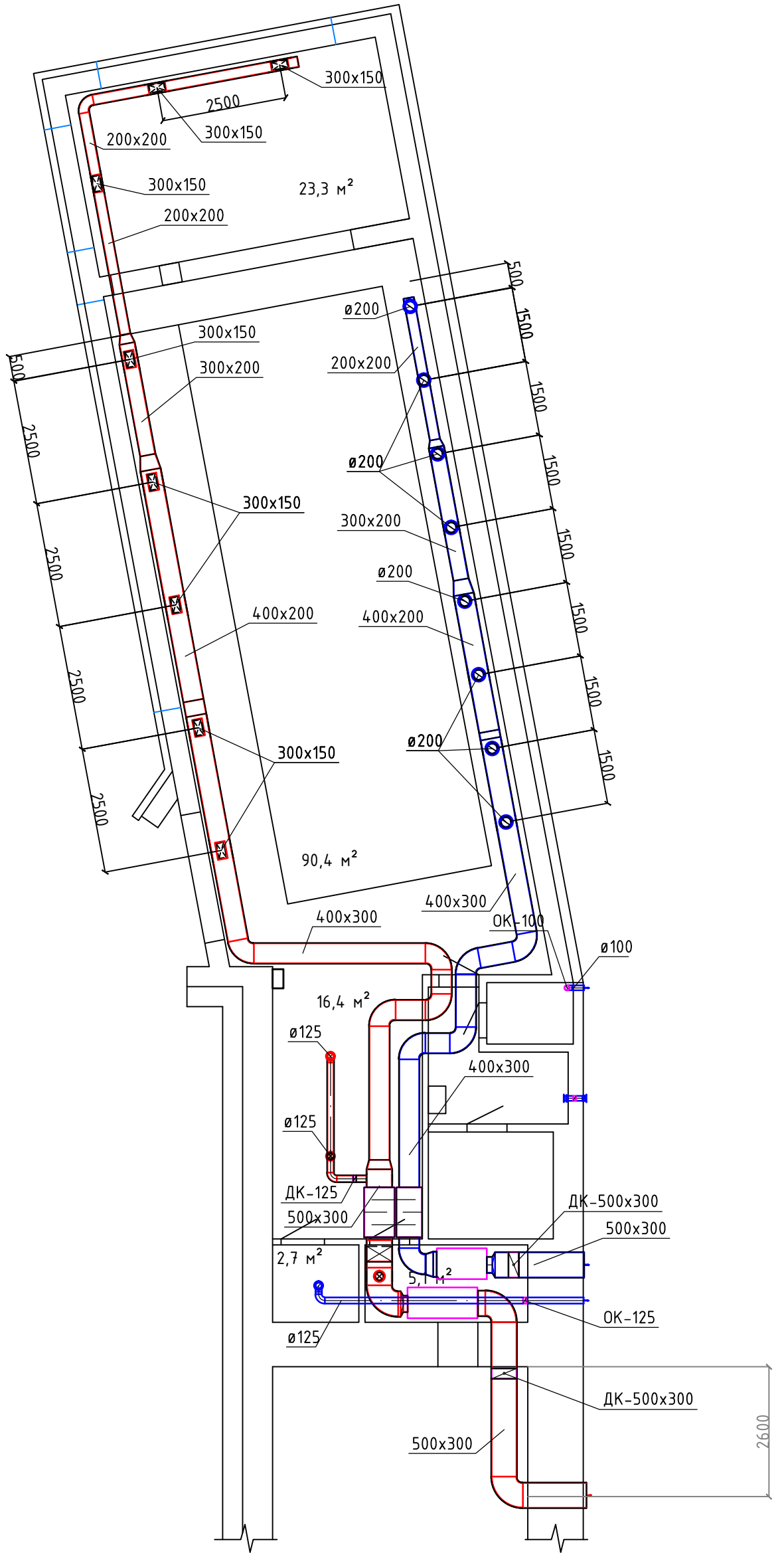
План 1 этажа
