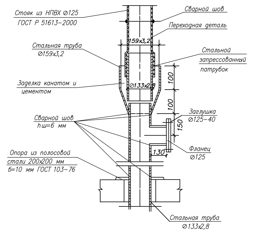
Узел "Б"
