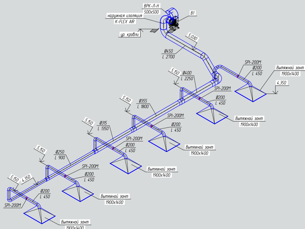
Схема системы
