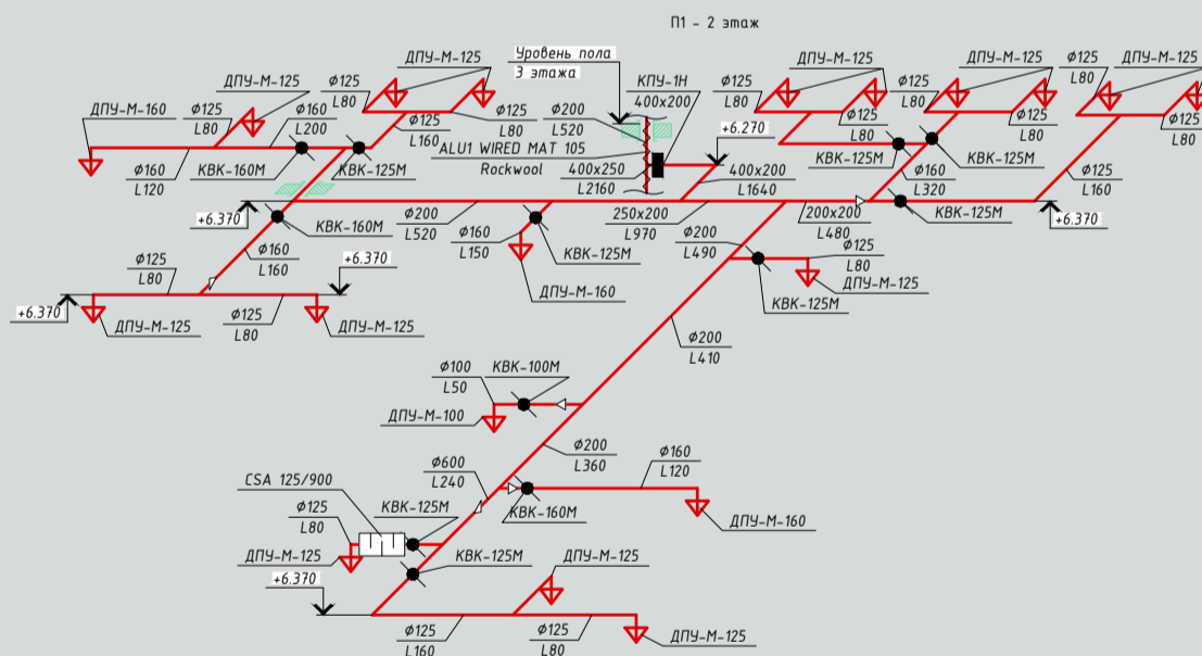
Схема системы вентиляции
