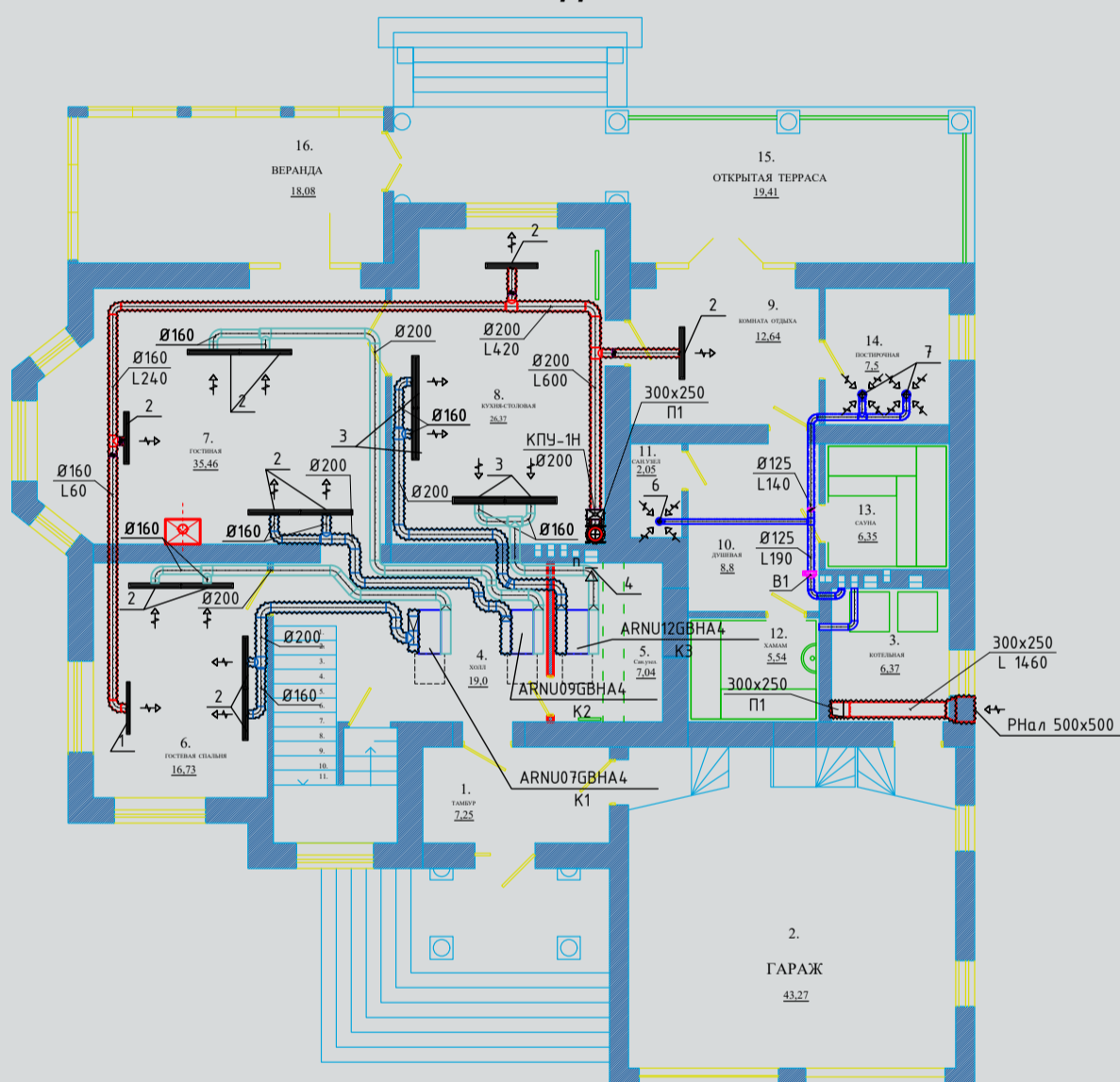
Схемы систем
