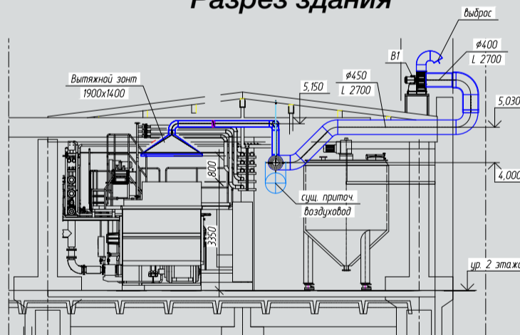
Схема системы
