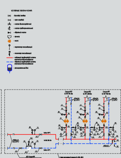
Тепловая схема
