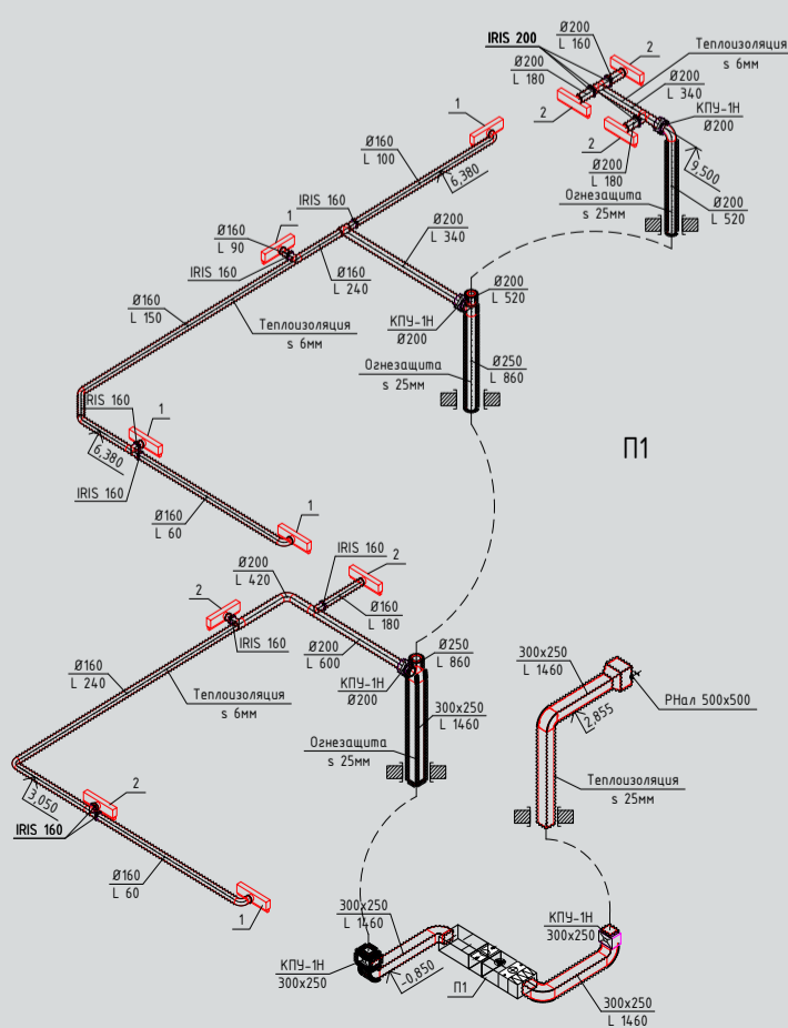
Схемы систем
