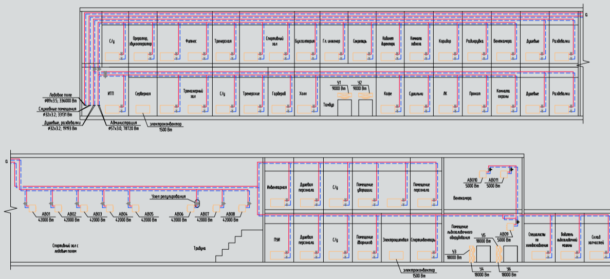
Принципиальная схема системы отопления
