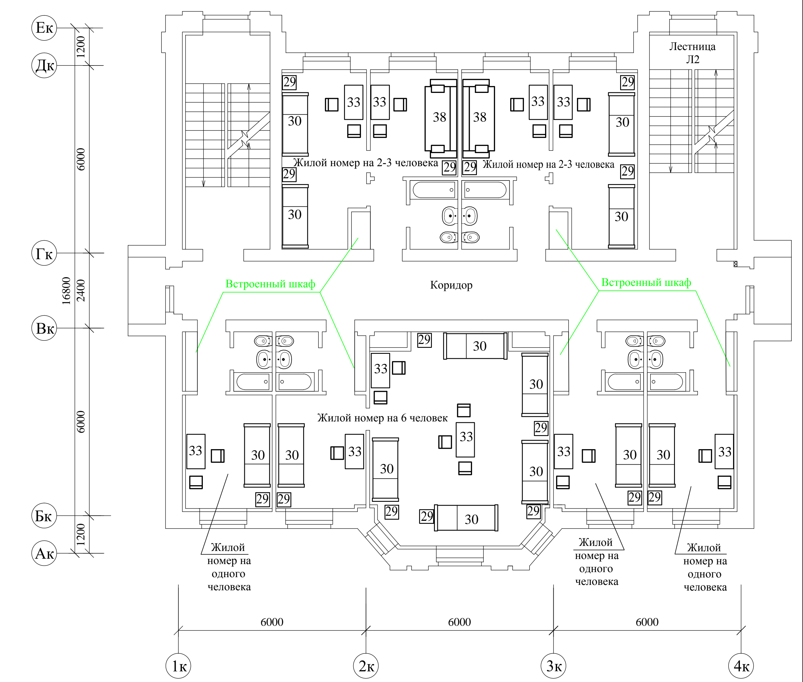
План на отм. +9,700
