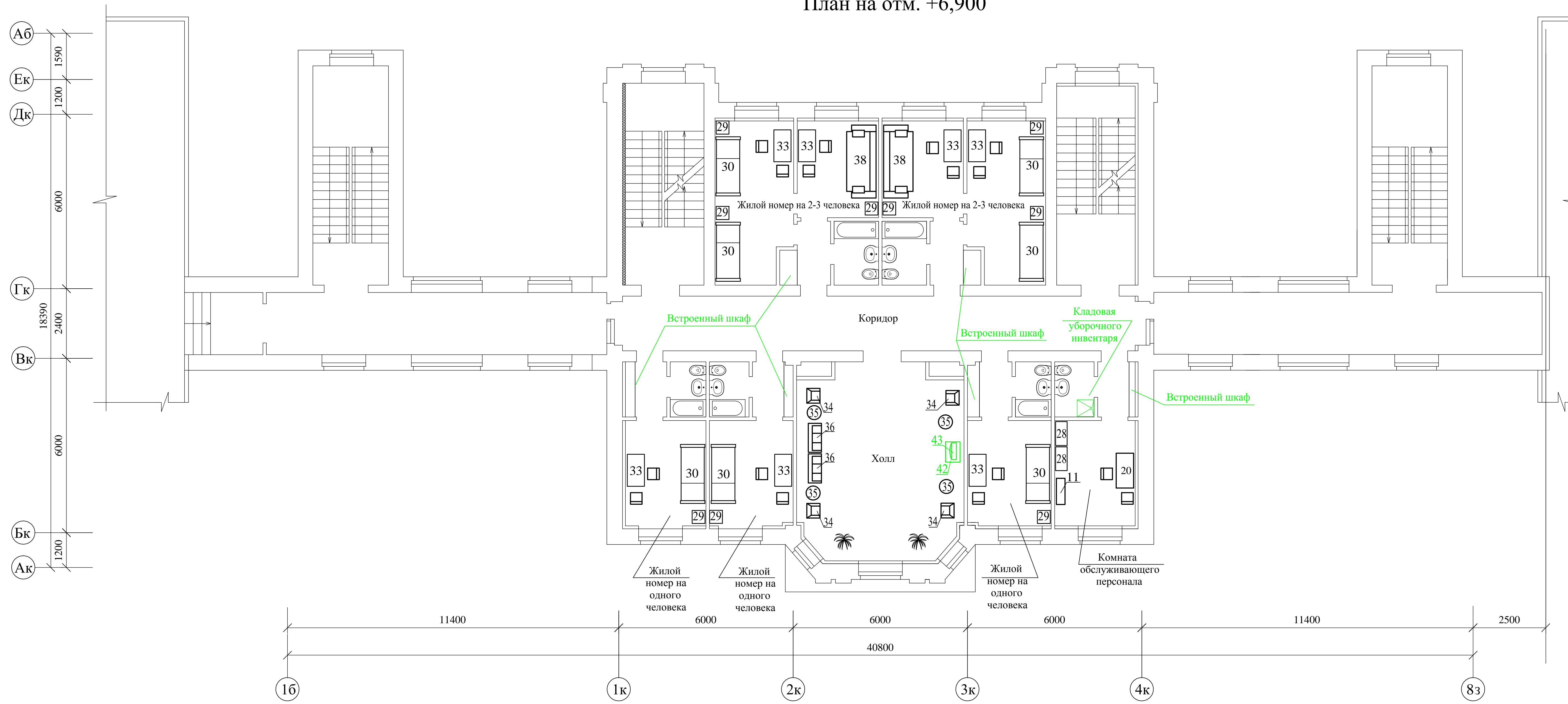
План на отм. +6,900
