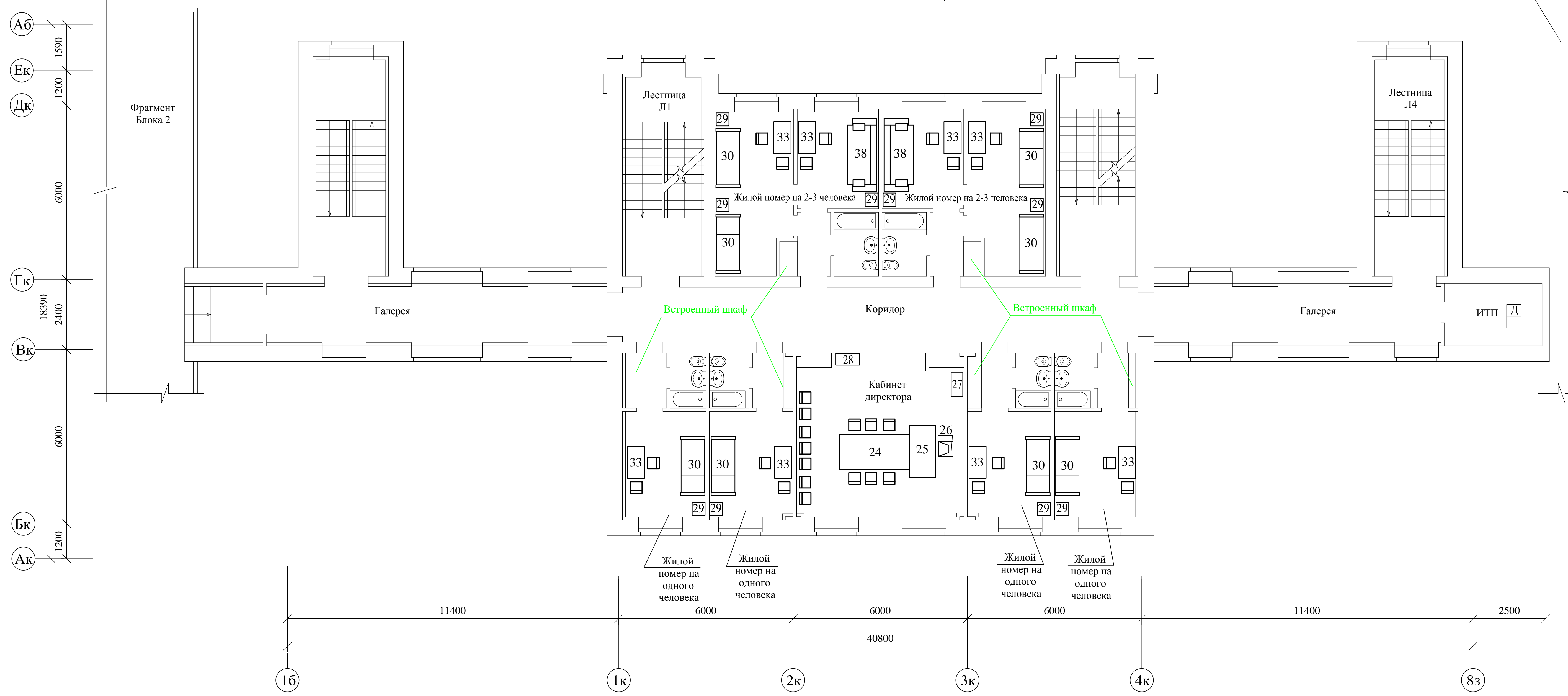
План на отм. +3,600
