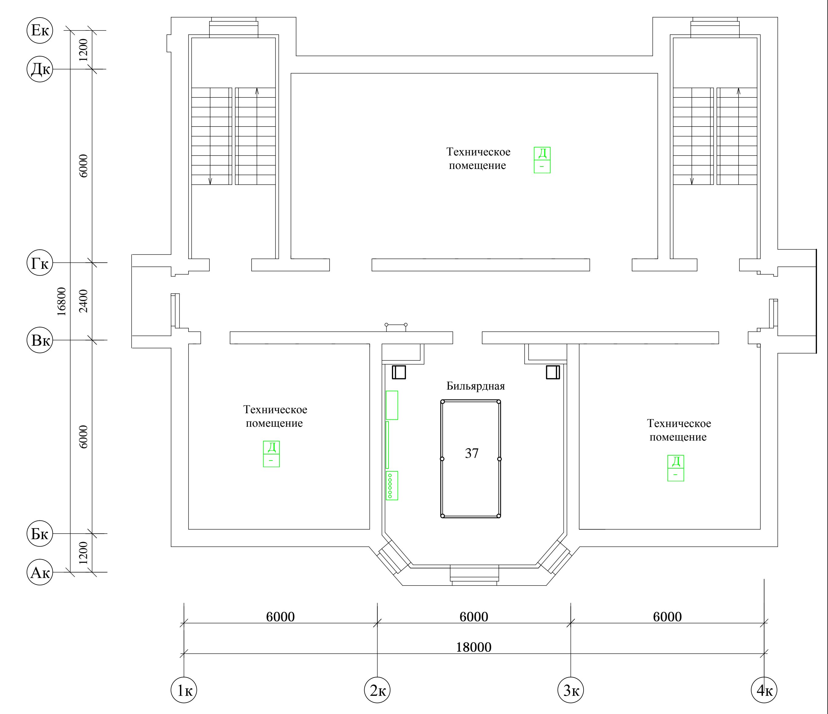
План на отм. +12,500
