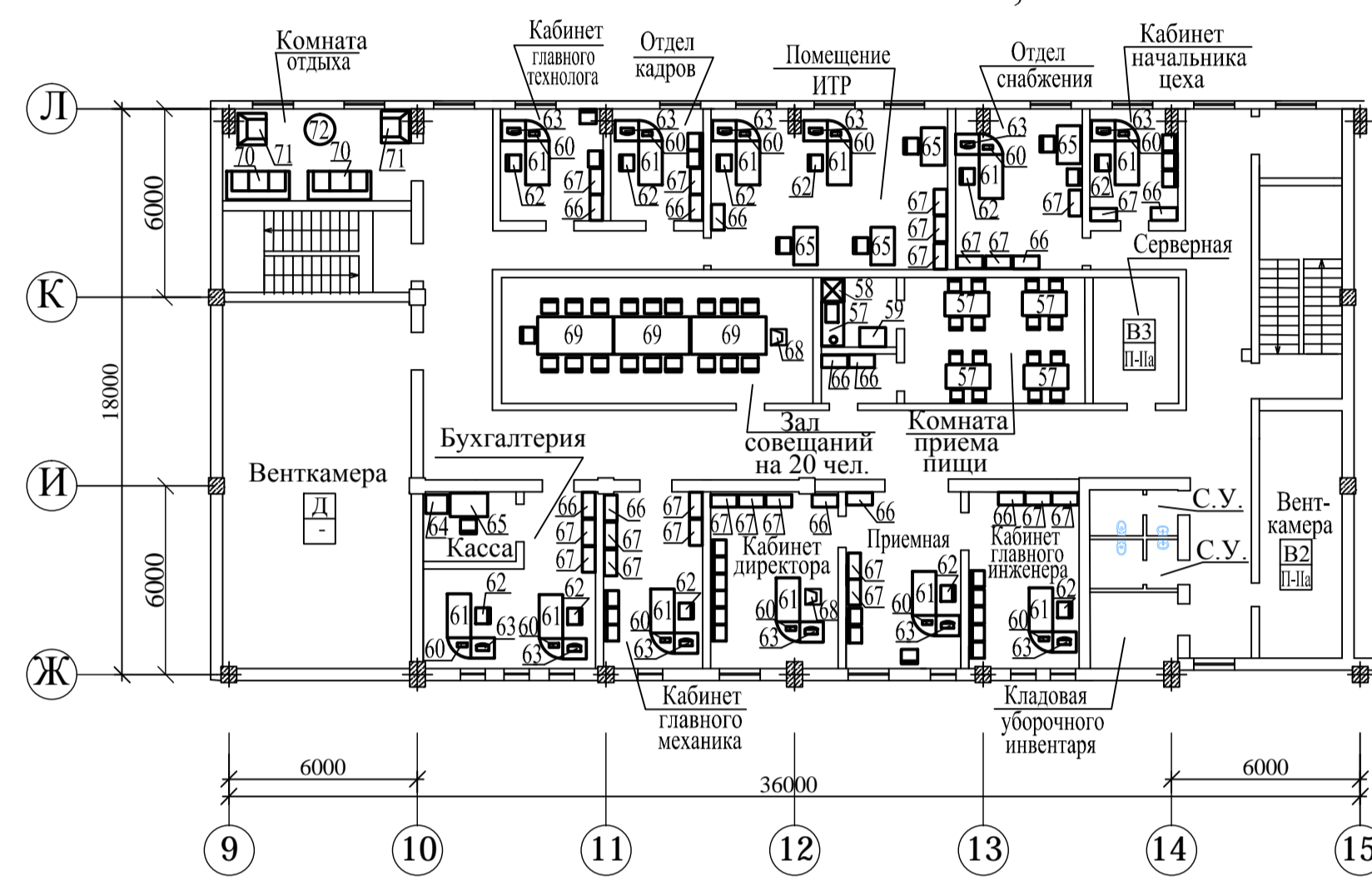
План на отм. +5,500
