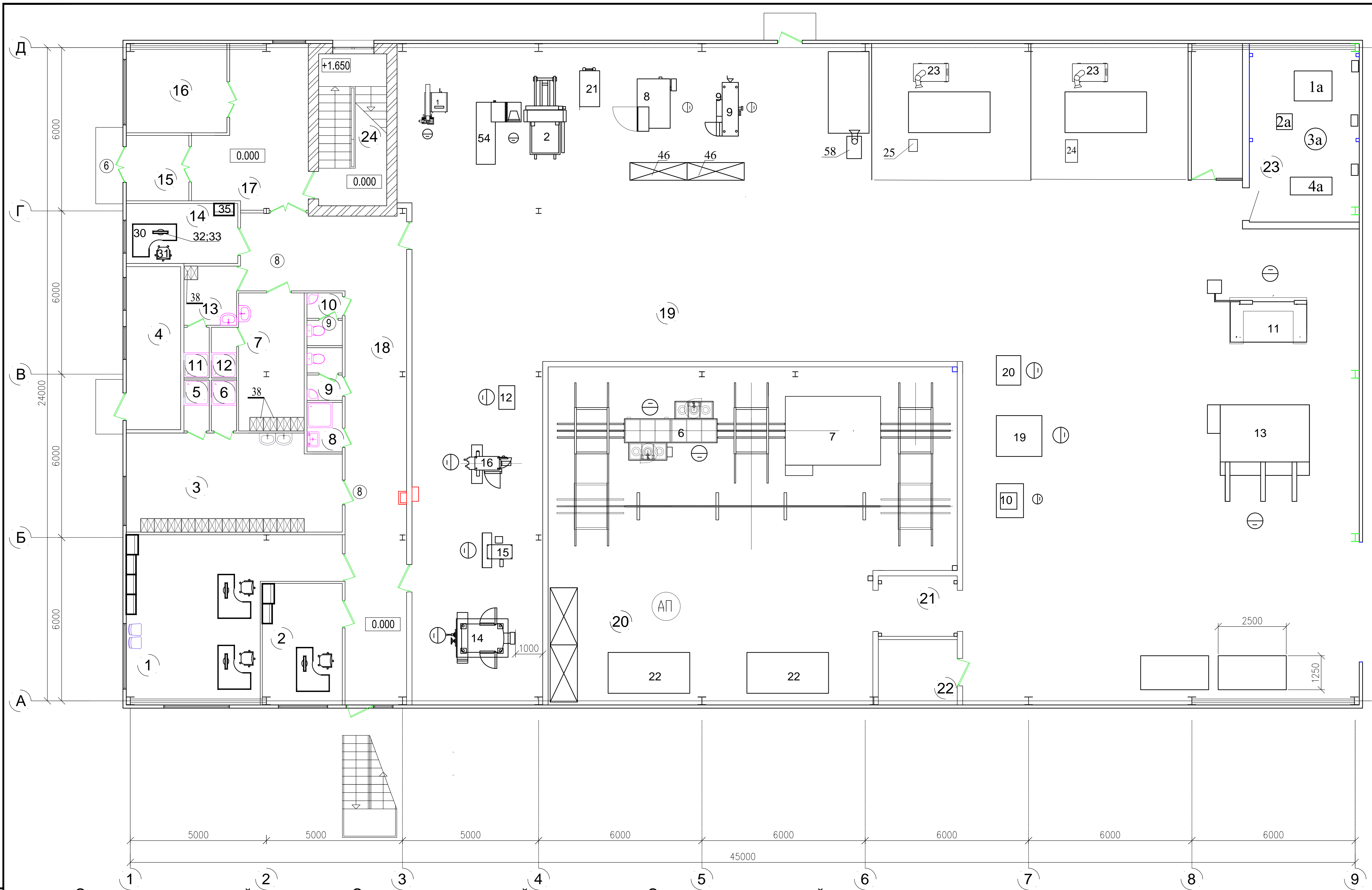
Экспликация помещений
