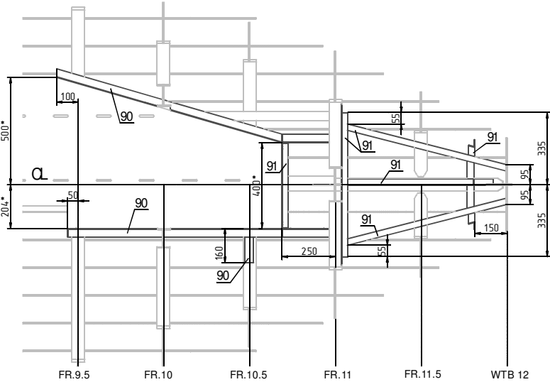
Сечение Ж-Ж
