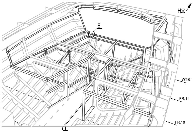
Изометрический вид каркаса носового салона (настил палубы и панели условно не показаны)
