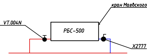
Подключение отопительного прибора
