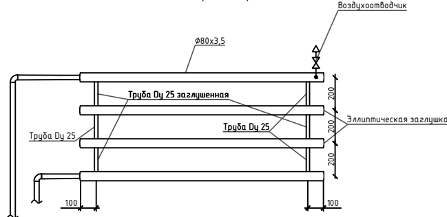
Узел подключения регистра
