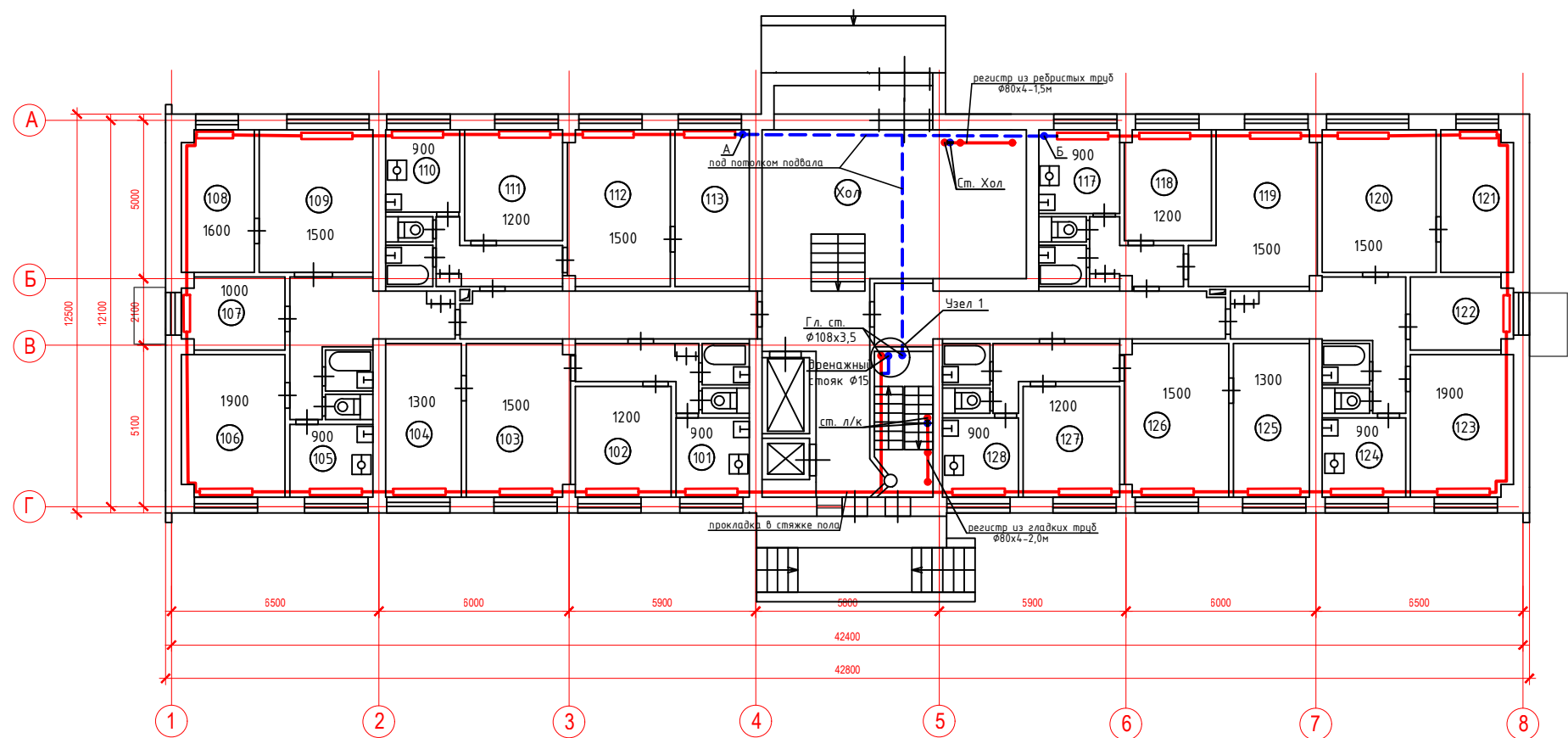
План 1-го этажа М 1:200
