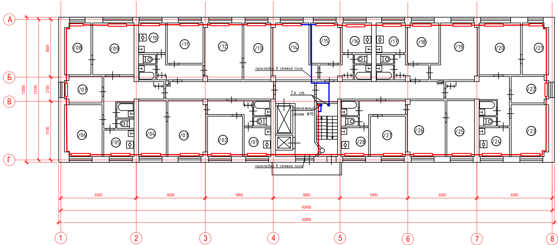
План типового этажа (2-16)
