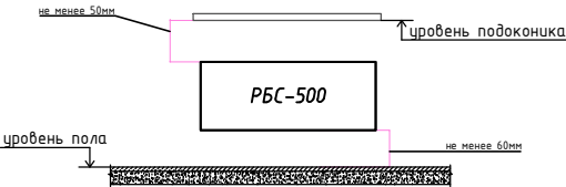
Установка отопительных приборов под окном
