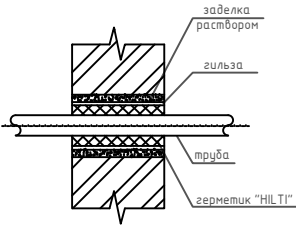
Прокладка трубопровода отопления через стены
