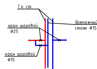
Узел 1. Подключение дренажного стояка
