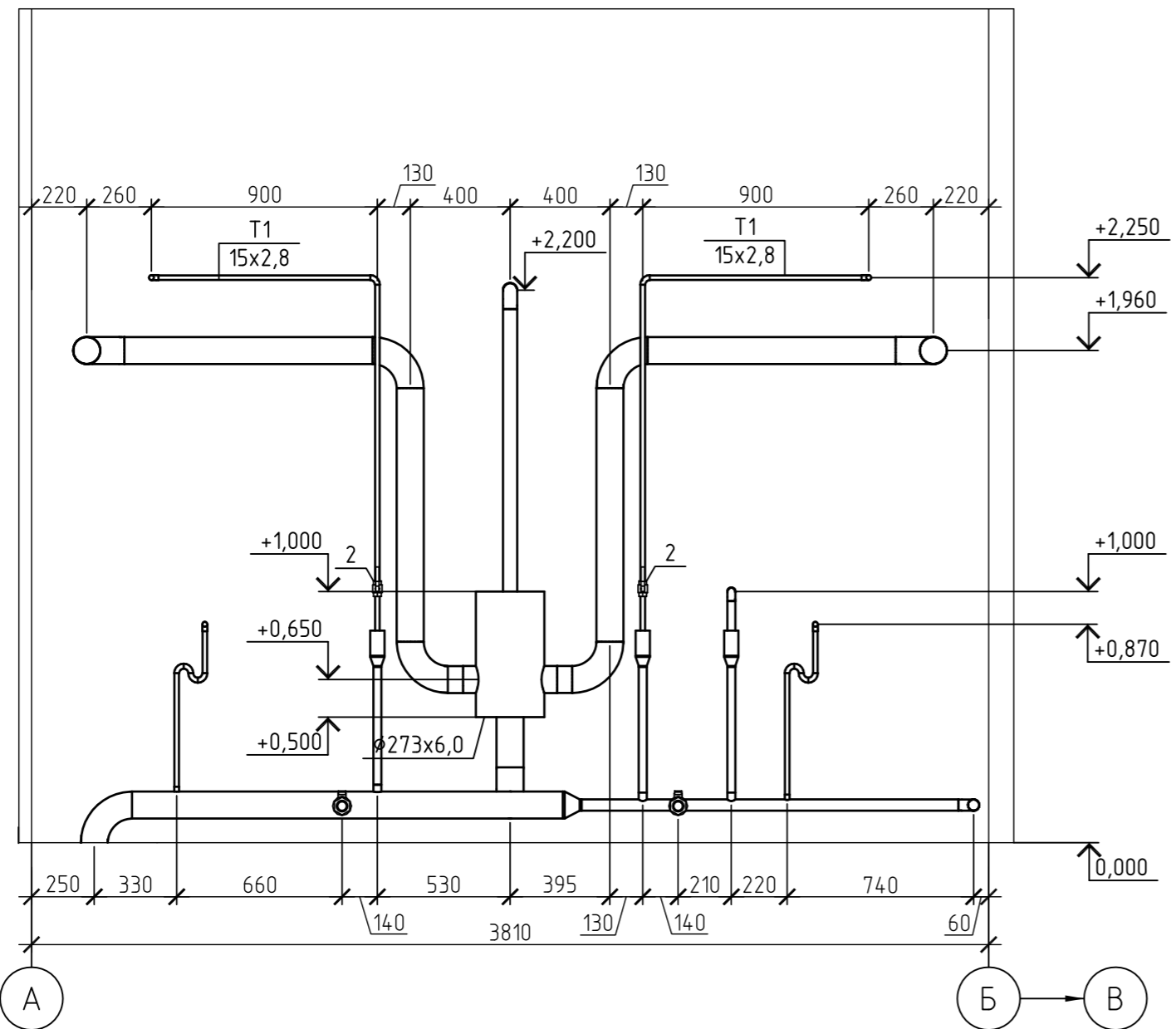
Разрез 1-1
