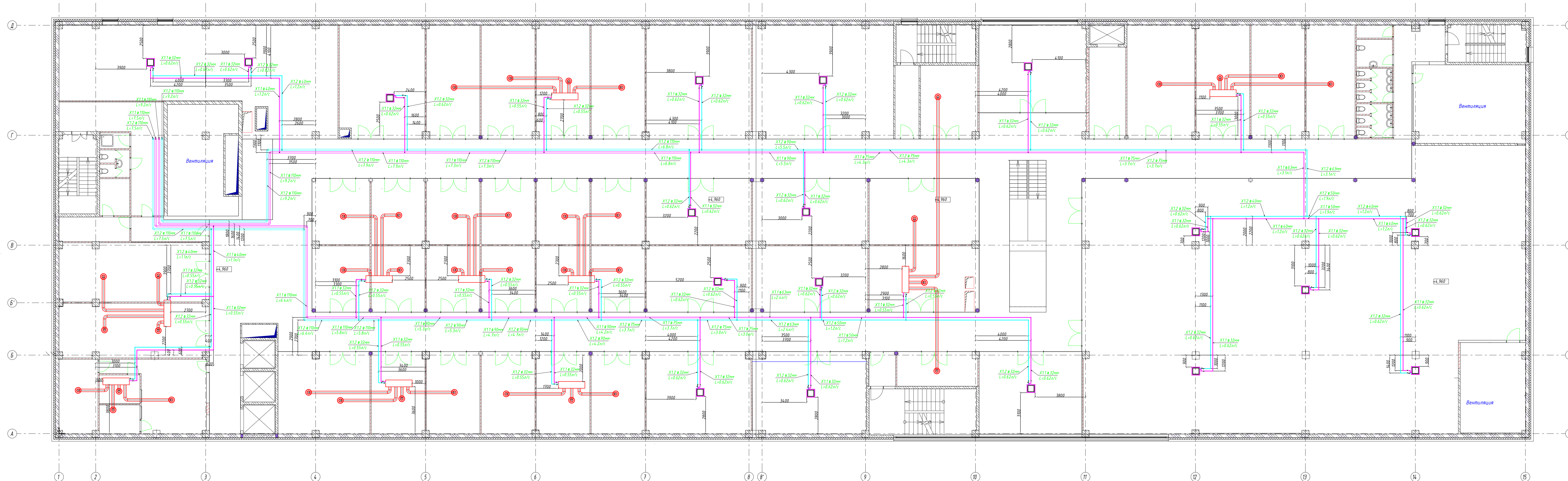
План 2-го этажа на отм. +4,950
