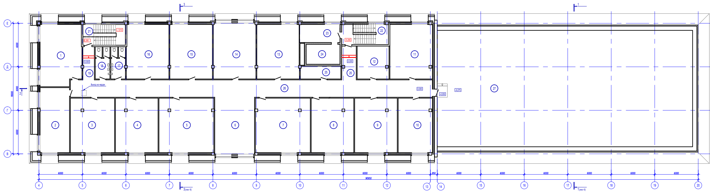
Экспликация помещений мансардного этажа(начало)
