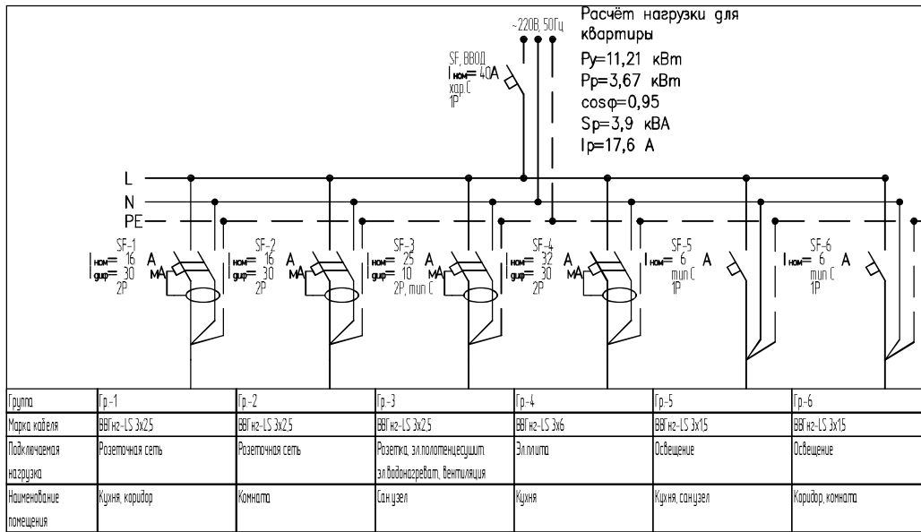
Щиток квартирный. Вид спереди (крышка корпуса не показана)
