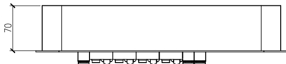
Щиток квартирный. Вид сверху (крышка корпуса не показана)
