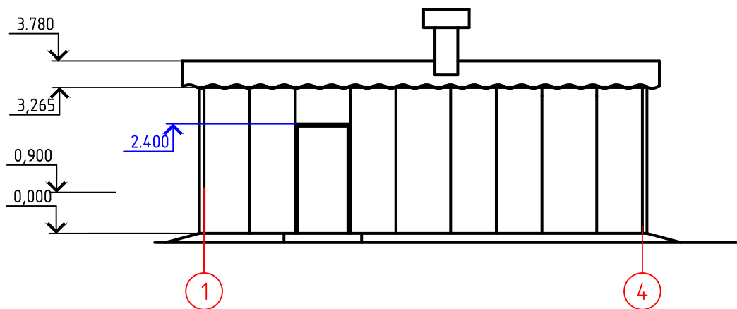
Фасад 1-4
