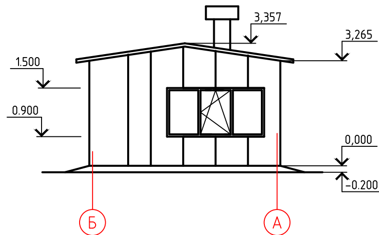
Фасад Б-А
