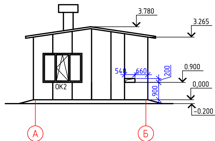
Фасад А-Б
