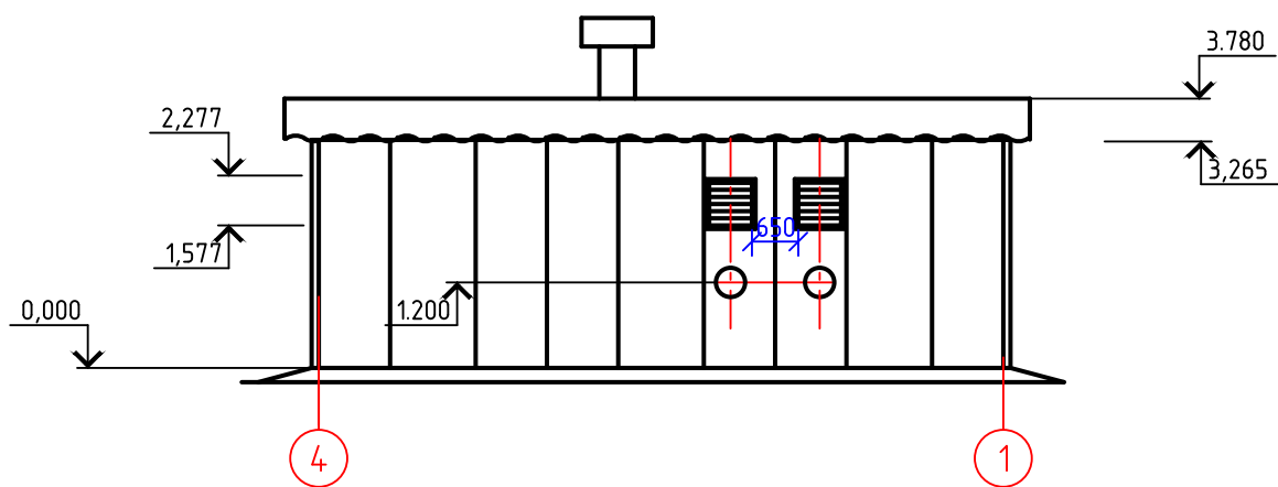
Фасад 4-1
