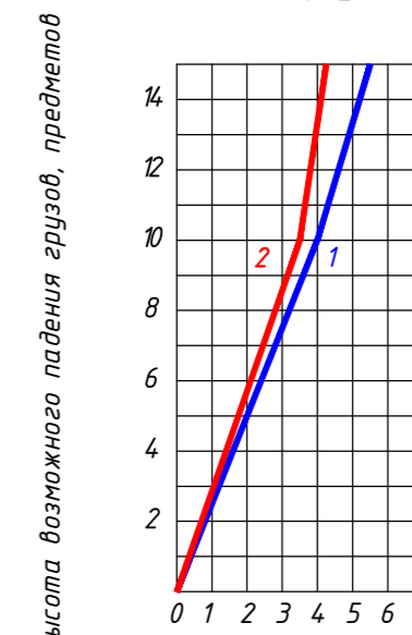
Минимальное расстояние отлета груза
