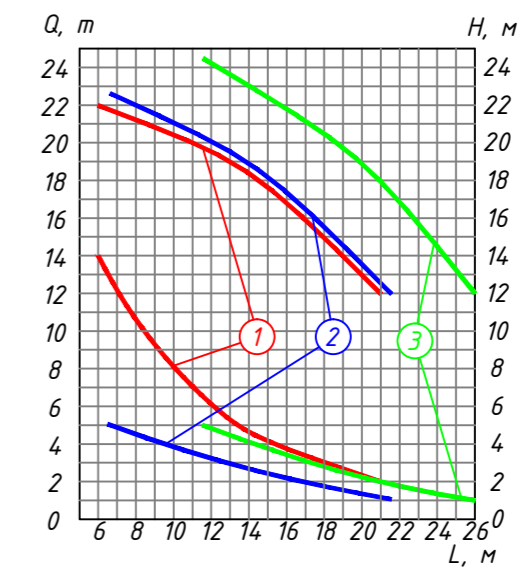
Грузовая характеристика гусеничного крана ДЭК-251 (Lстр=22,75 м; Lгус=5,00 м)
