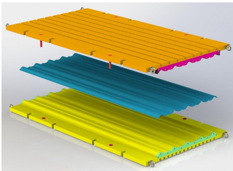
Штамповая оснастка
