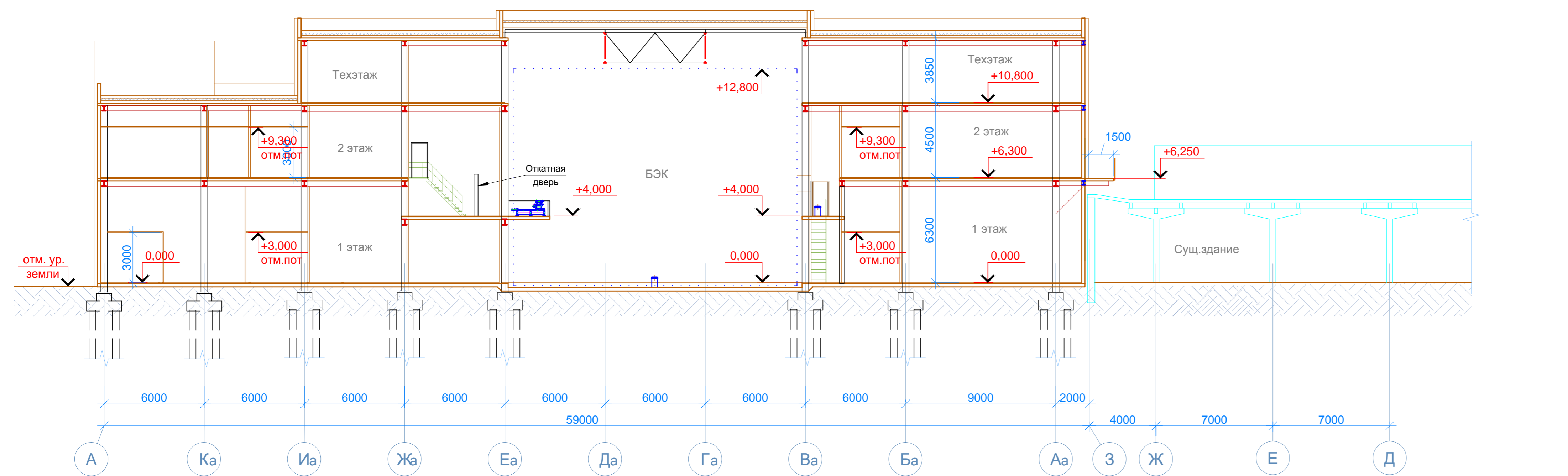
Разрез 1-1
