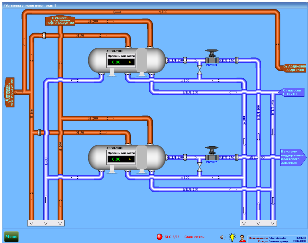
рис. 3.3.2 Мнемосхема АГОВ.
