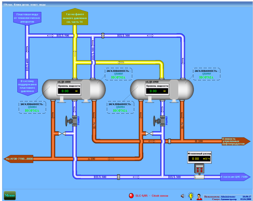
рис. 3.3.1 Мнемосхема АБДВ.
