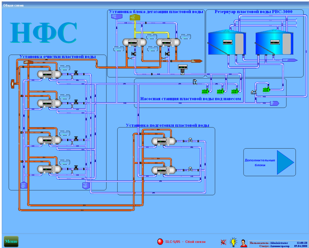
рис. 3.3 Общая схема.
