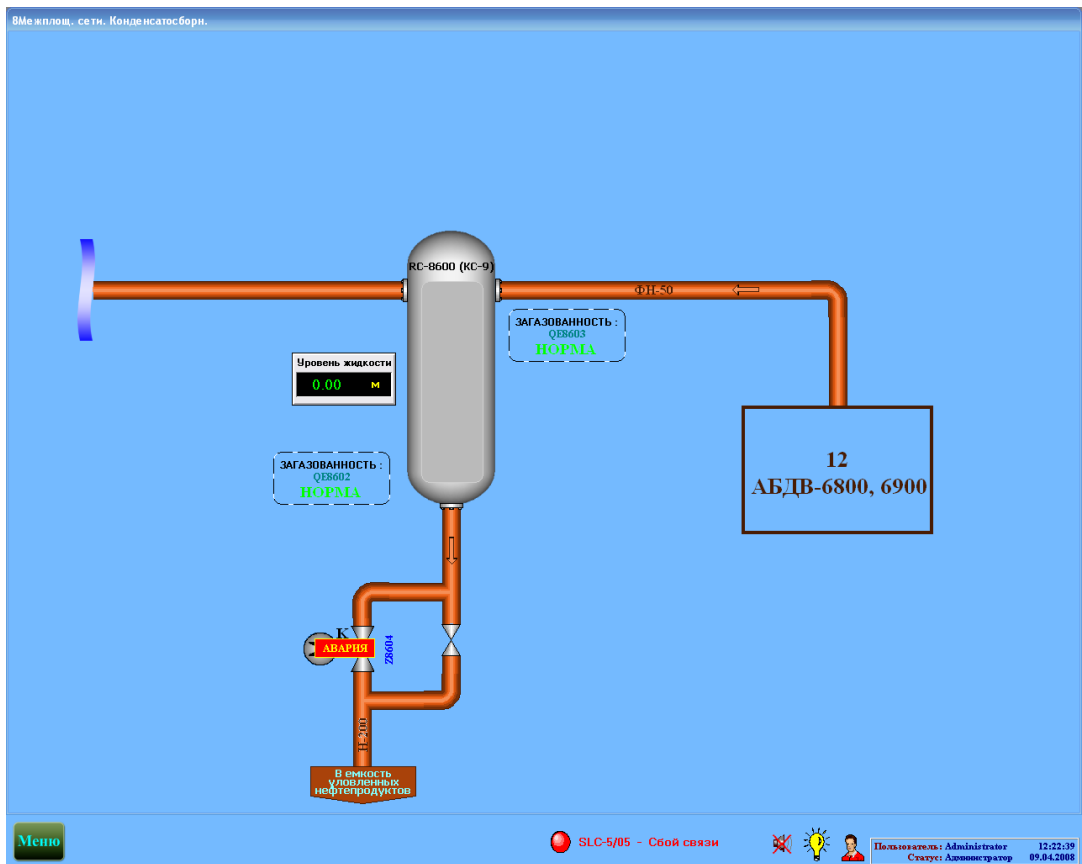
рис. 3.3.3 Мнемосхема Межплощадочные сети. Конденсатосборники.
