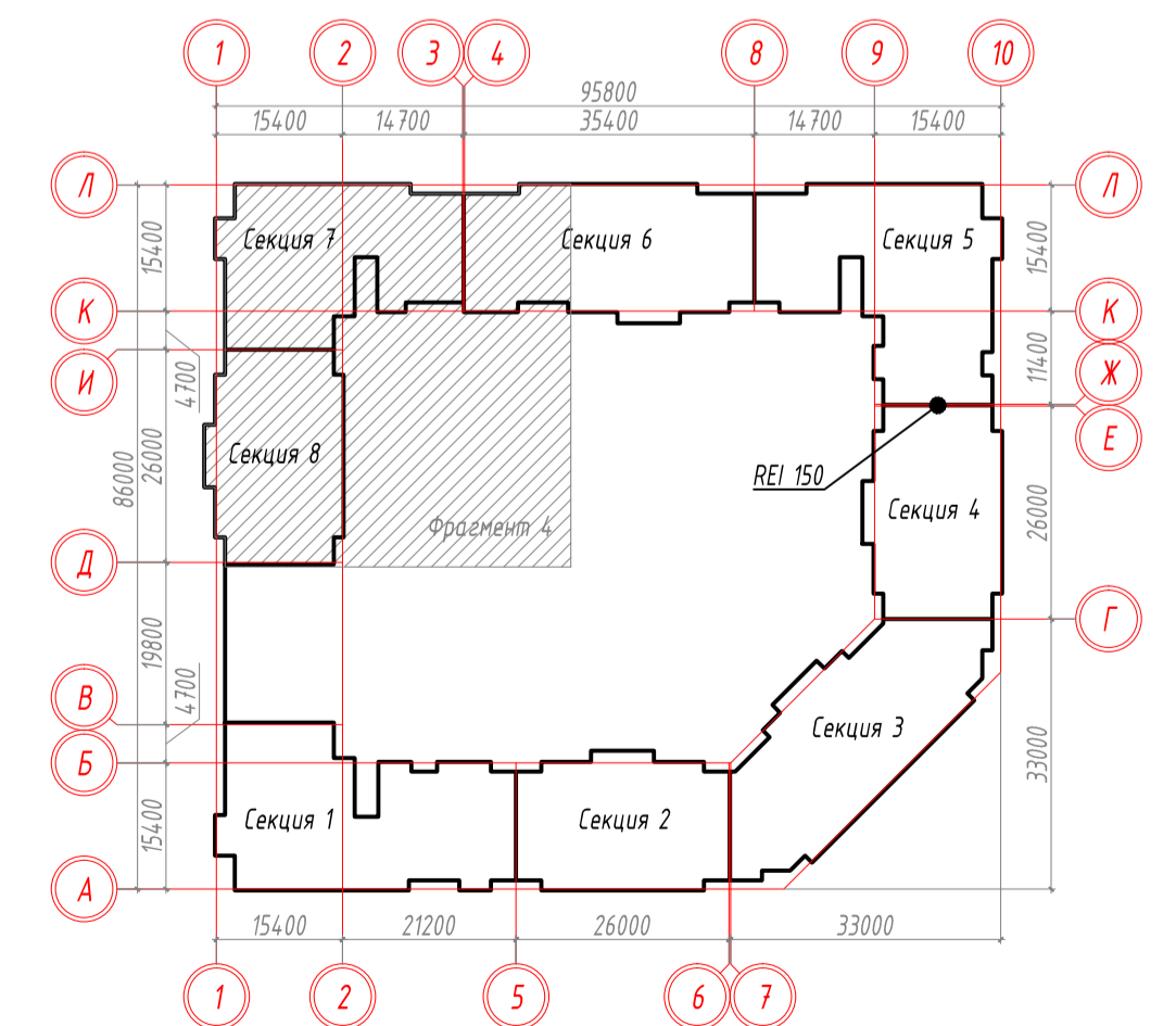
Компоновочная схема
