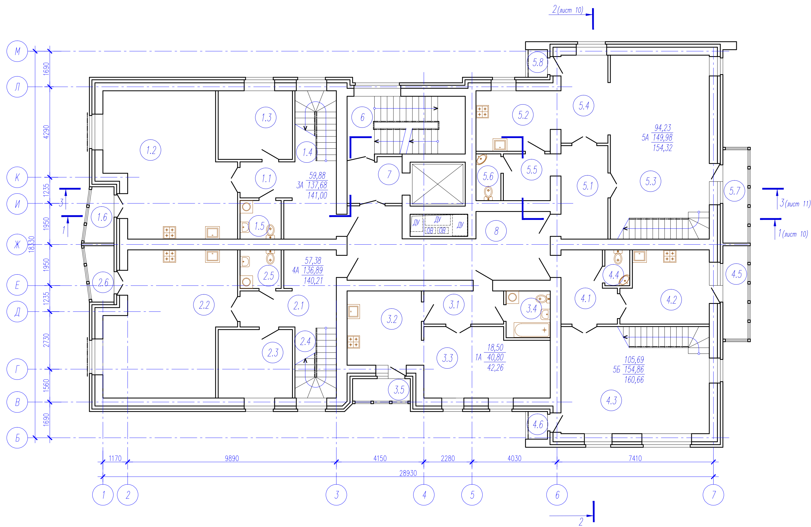
Экспликация помещений девятого этажа (начало)
