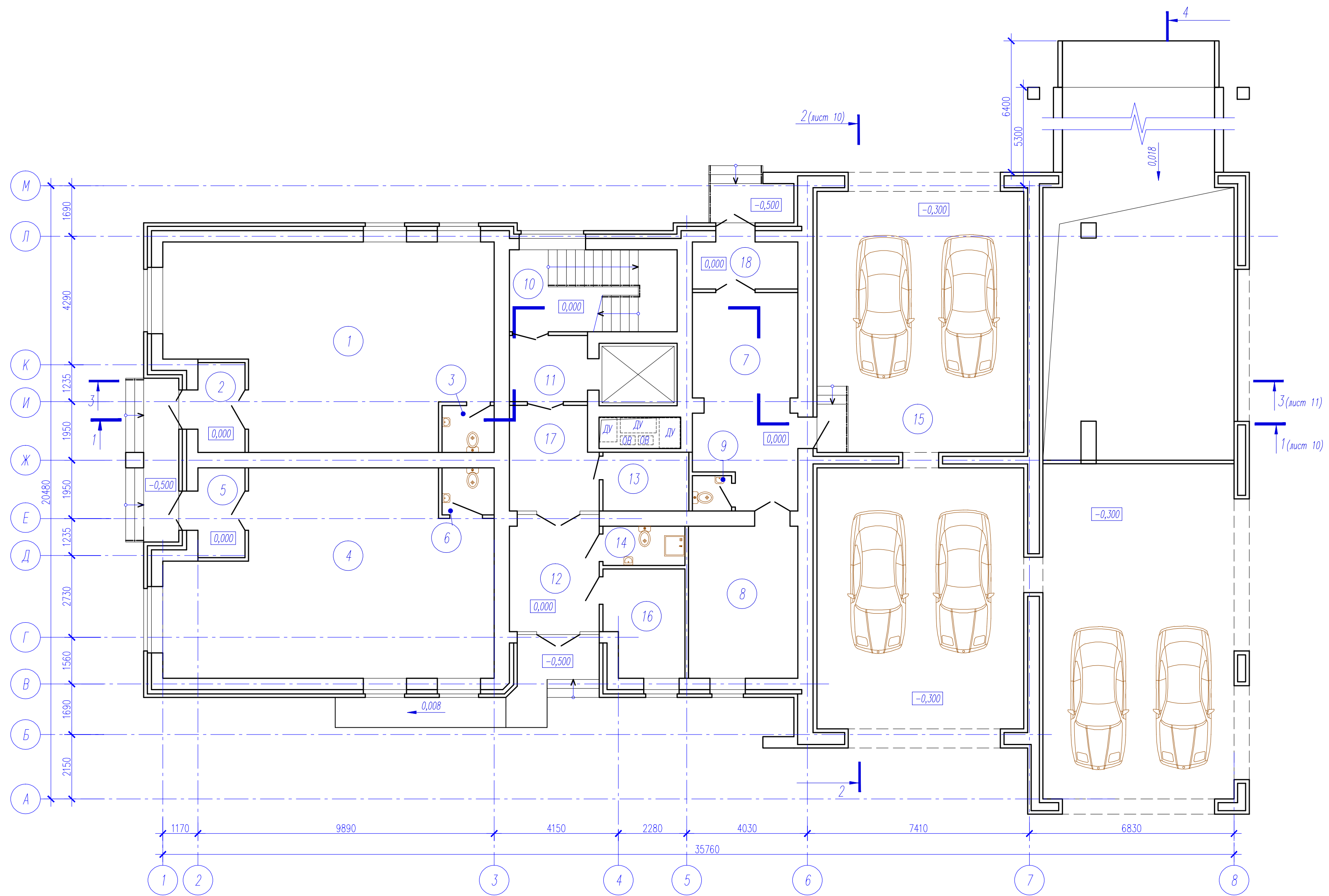
Экспликация помещений первого этажа (начало)
