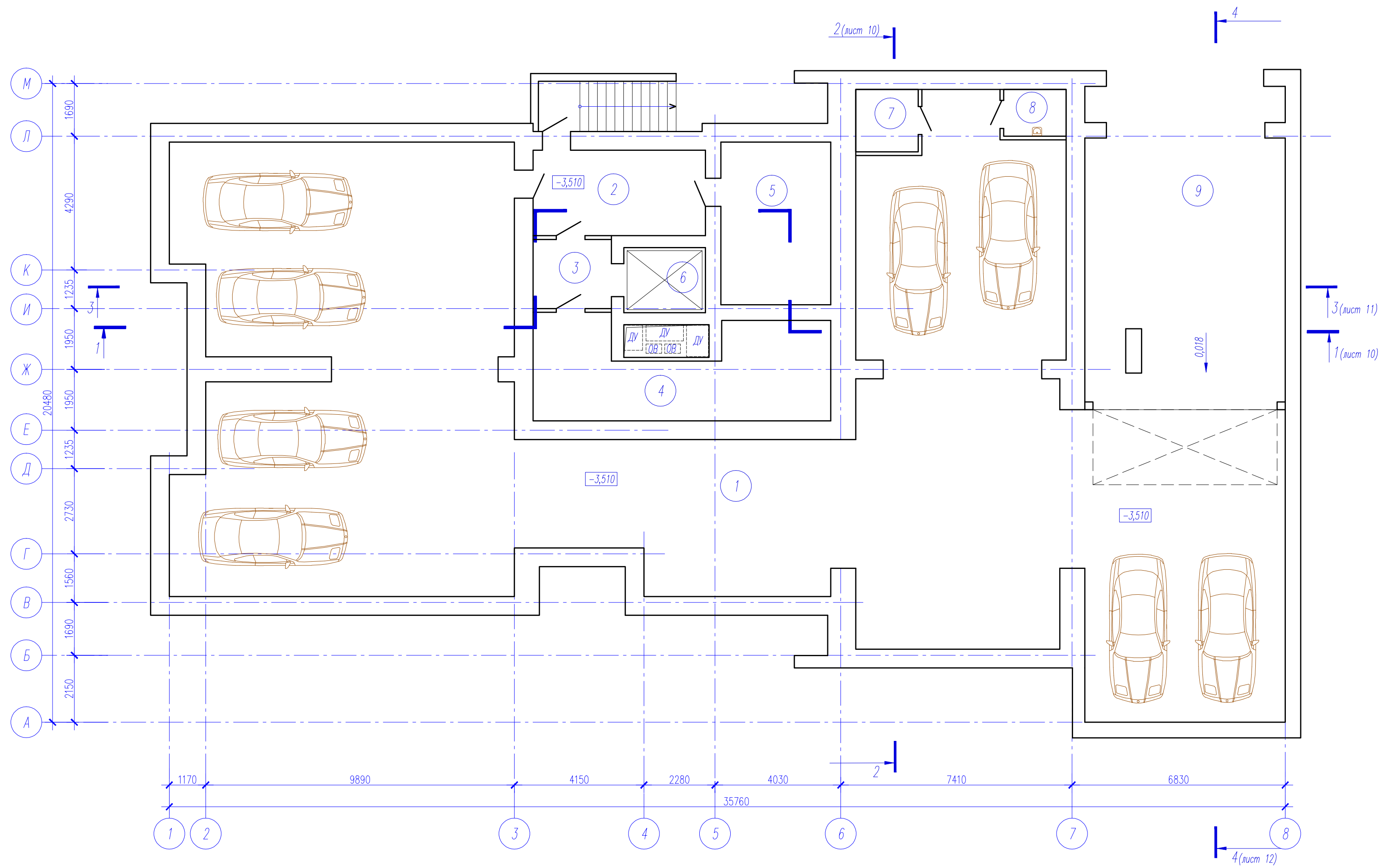
Экспликация помещений подвального этажа
