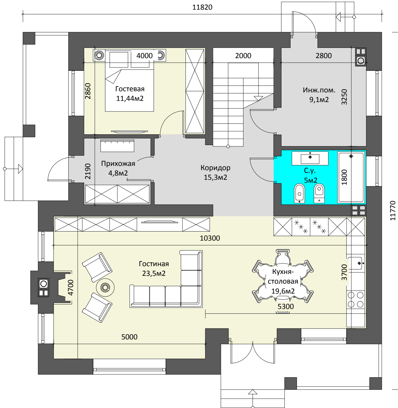
ПЛАН 1 ЭТАЖА 5 помещений этажа = 88,74м²
