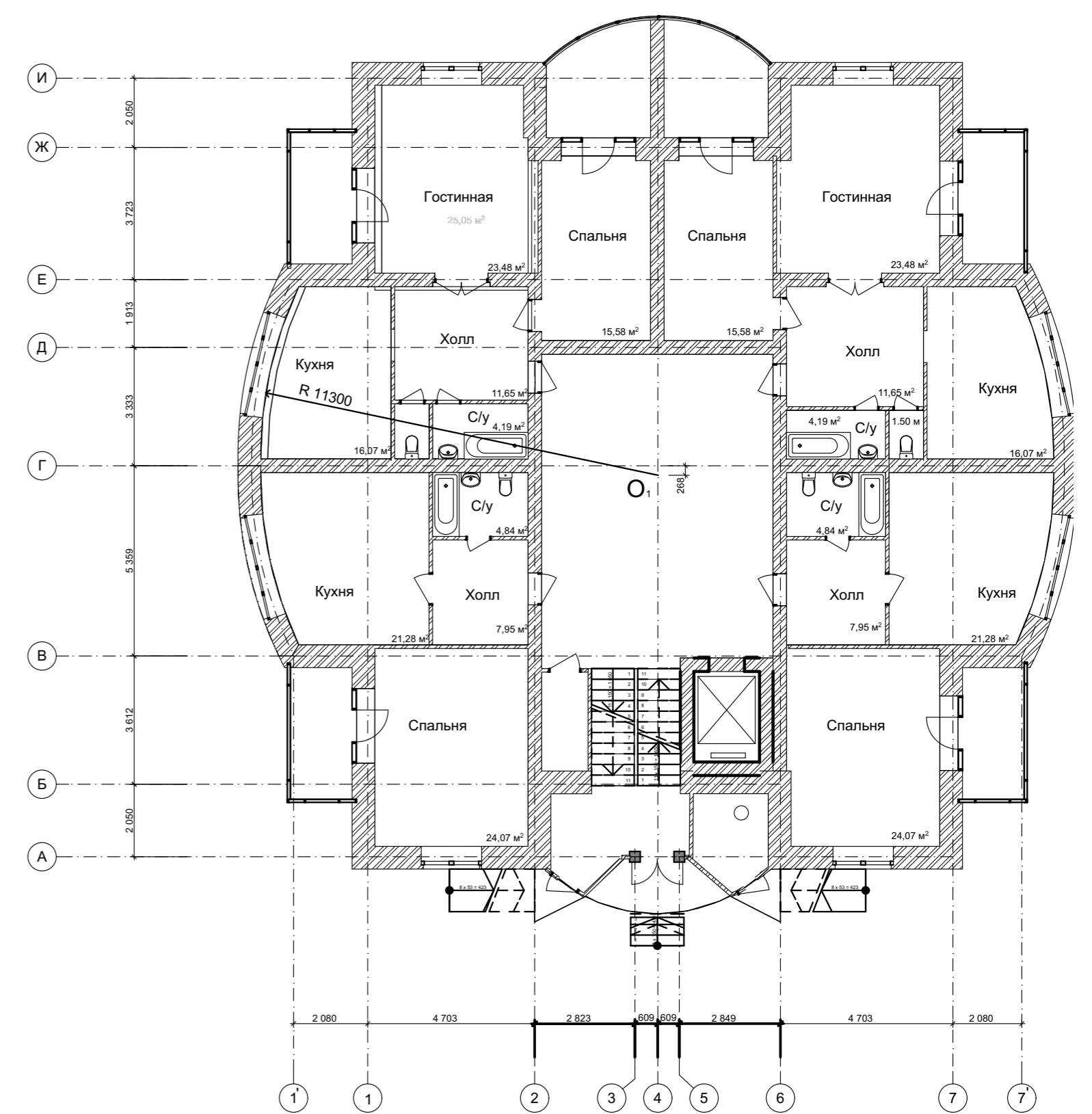
План 1-го этажа М1:200
