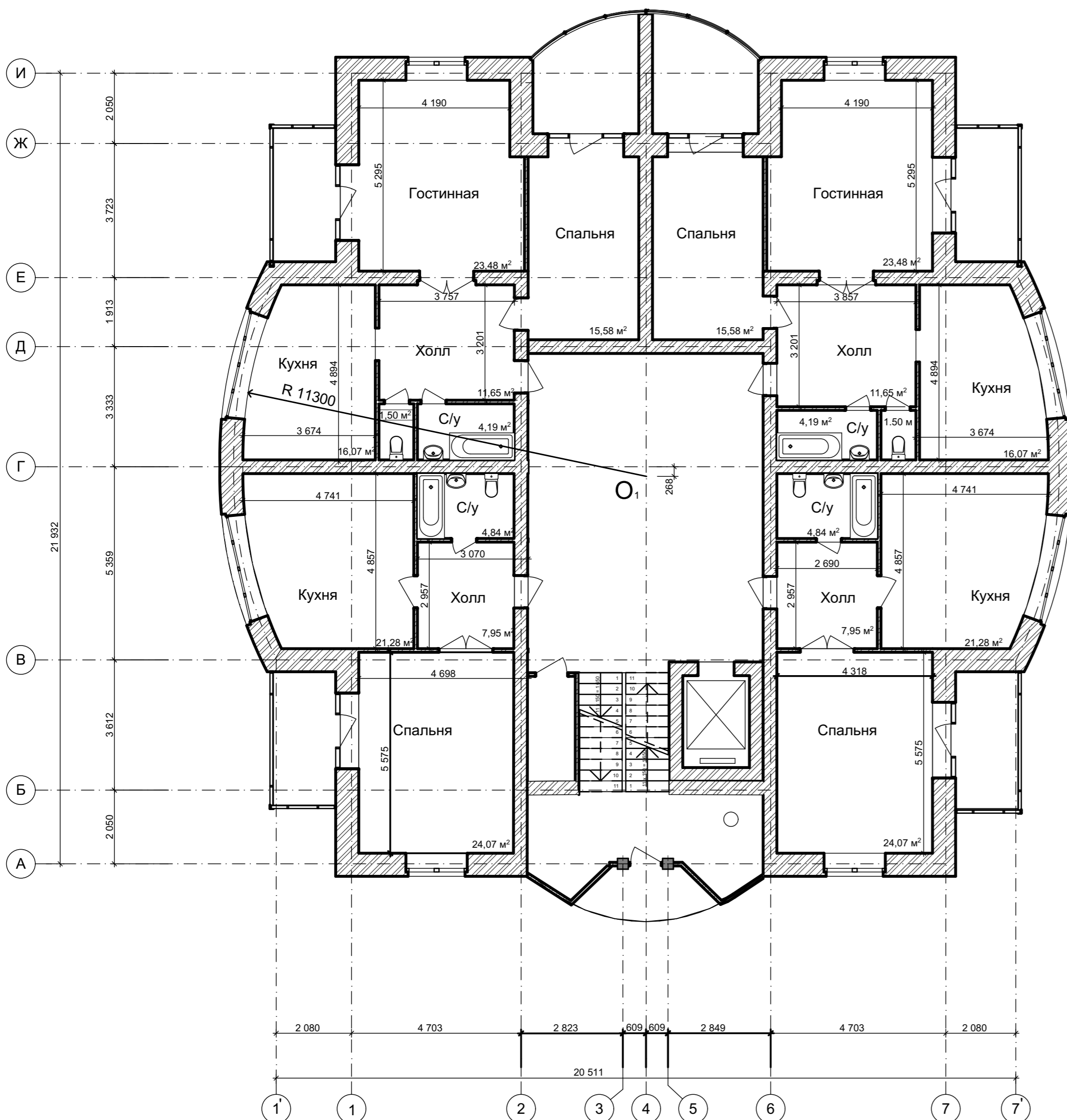
План типового этажа М 1:100
