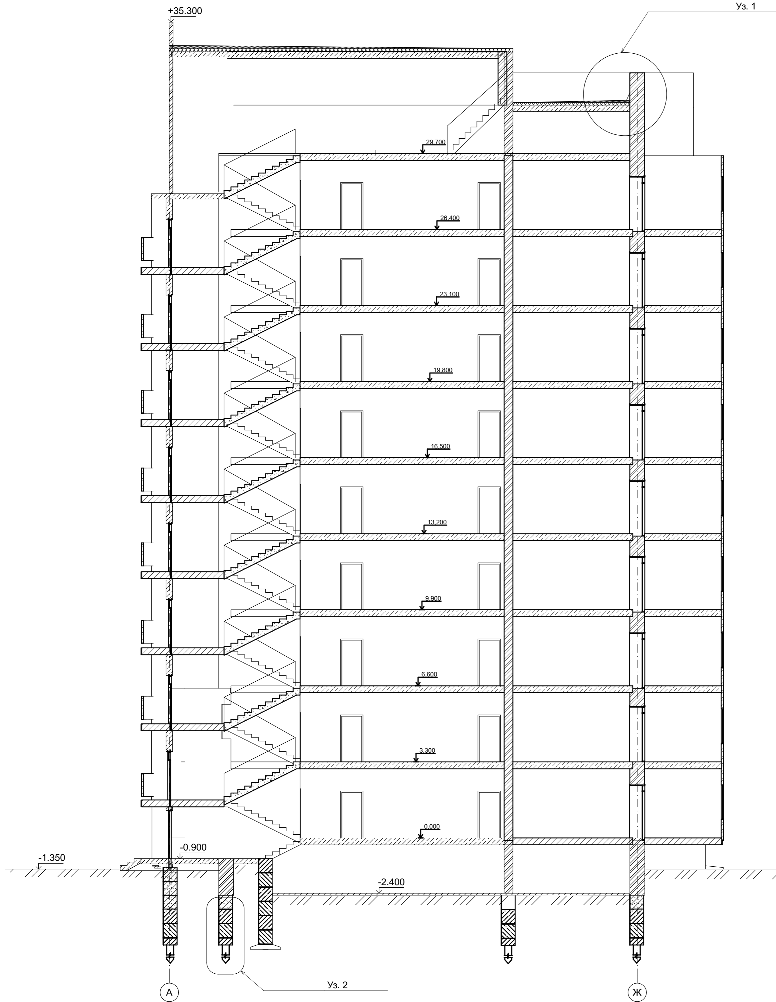
Разрез 1-1 М 1:100
